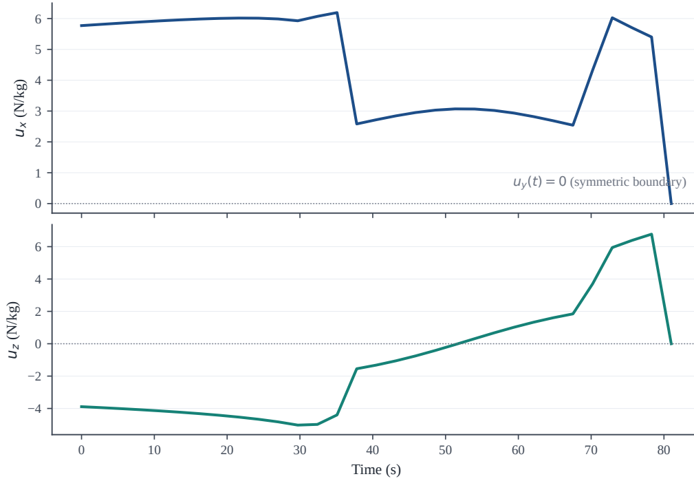
图 11 非零控制加速度分量 u_x 、 u_z 的时间演化曲线；对称边界使 u_y 全程为零。
