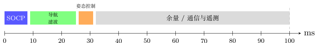
图 12 制导周期时间预算分配 (100 ms 周期)
