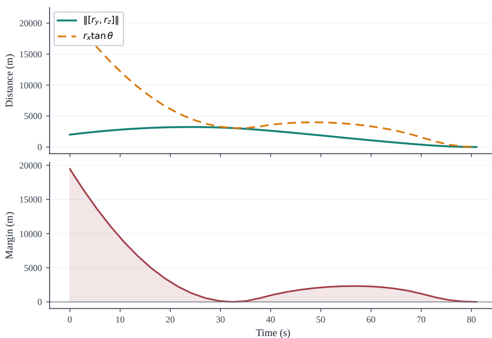
图 7 下滑角约束验证。上: \|[r_y, r_z]\| 与 r_x \tan \theta 对比；下: 约束余量。
