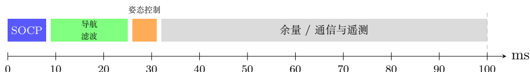
图 13 制导周期时间预算分配（100 ms 周期）
