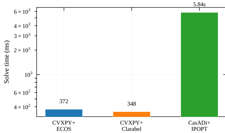
图 10: 各求解方案的单次求解耗时对比 (对数坐标)。C 手写版约 8 \mu\text{s} , Python 版约 350 \text{ ms} , IPOPT 约 5.8 \text{ s} 。
