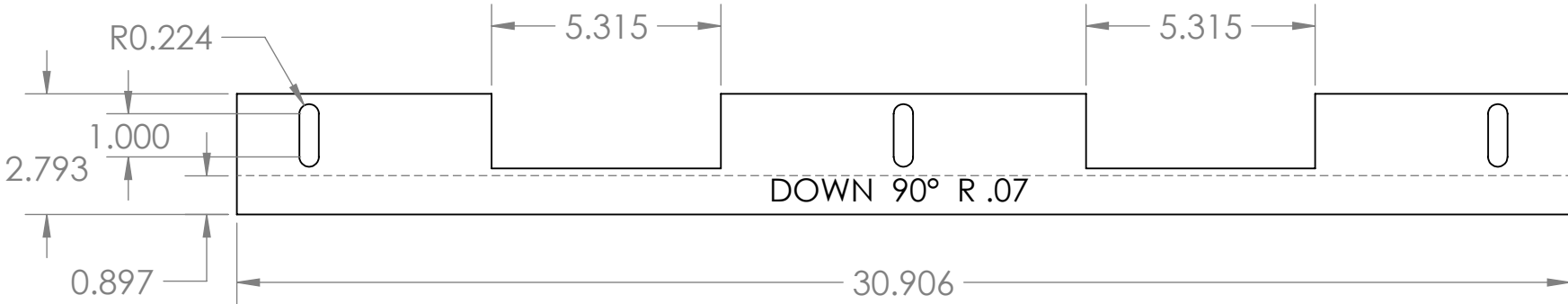
DET A
