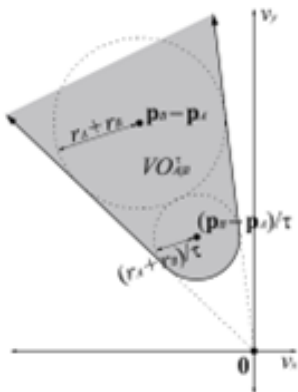
(a) 速度障碍集合
