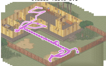
claude-fable-5.1
