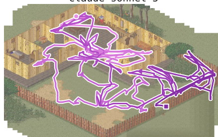
claude-sonnet-5
