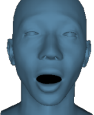
\rho = 2.0
