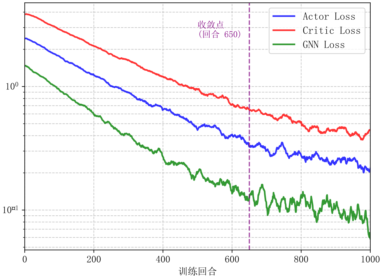
损失函数值 (对数尺度)
