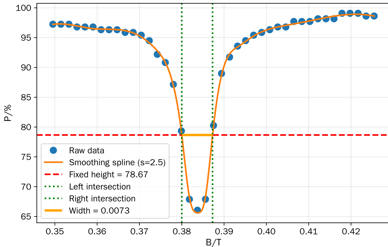
磁共振吸收曲线1
