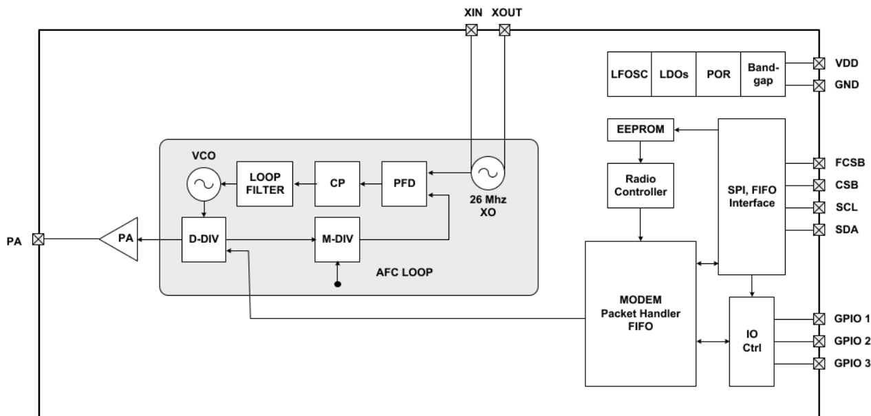
图 4-1. 功能系统框图
