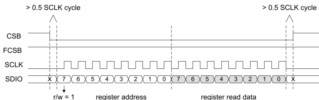
图 5-1. SPI 读寄存器时序
