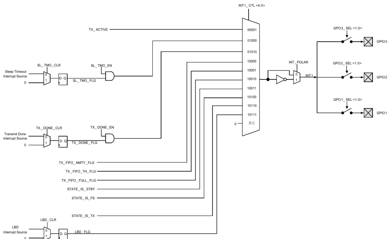
图 11. CMT2119B INT1 中断映射图
