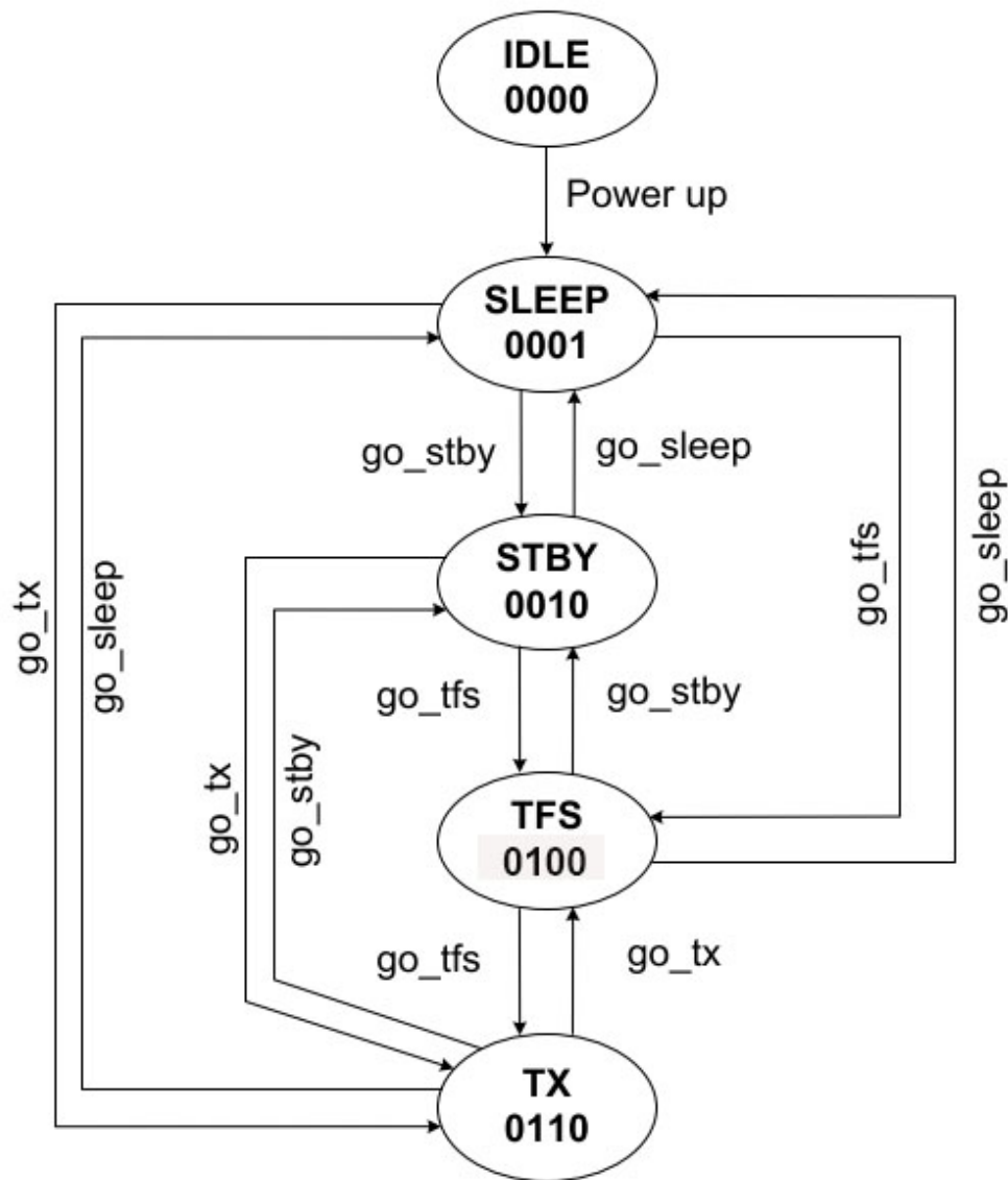
图 10. 状态切换图
