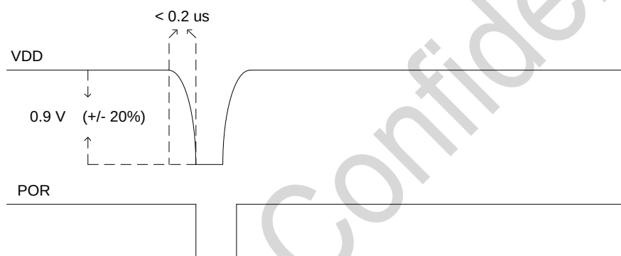
图 4-3. 电源电压迅速下降导致 POR 复位
