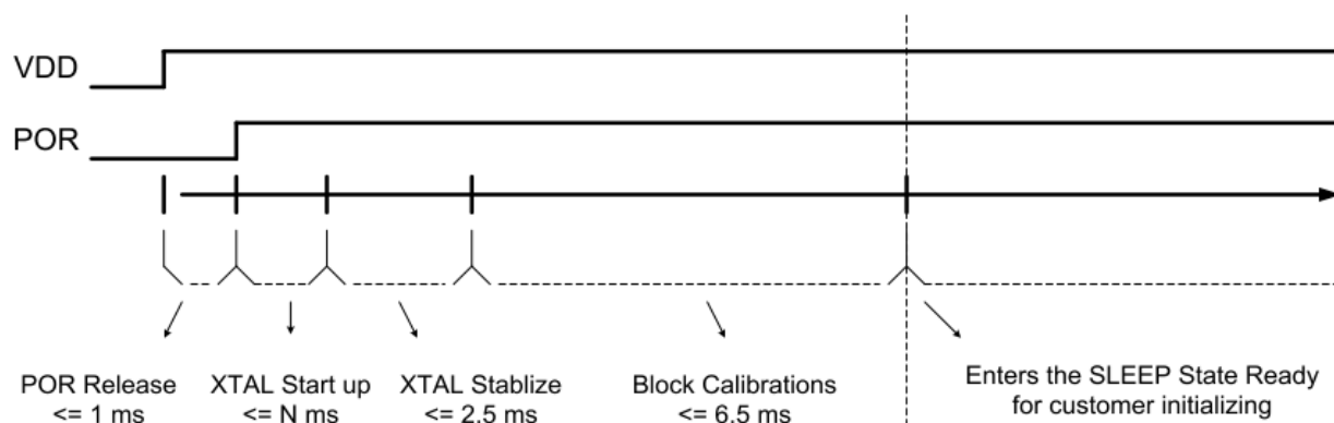
图 9.上电时序
