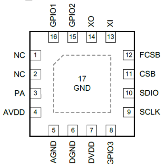
图 1. CMT2119B 管脚排列
