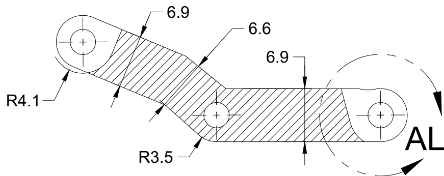
SECTION AK-AK
