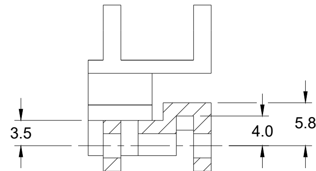
SECTION V-V
