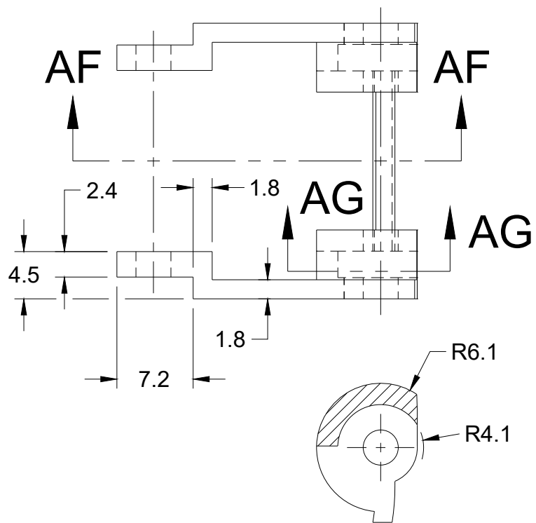
SECTION AG-AG
