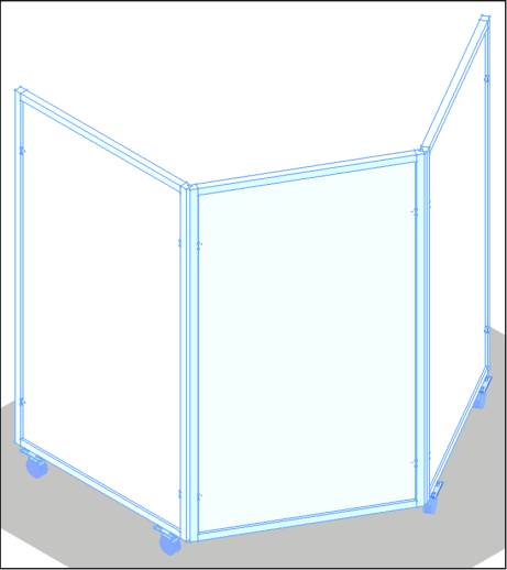
ISOMETRICA (1:25, mesma escala das vistas)
