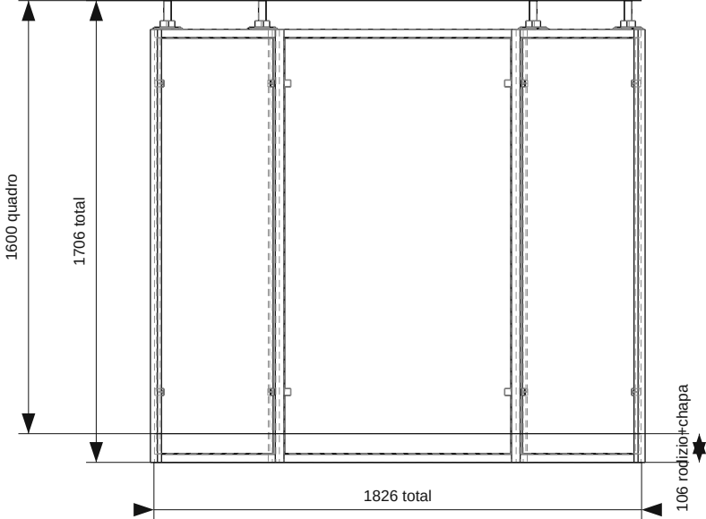
FRENTE (1:25), folha central de face
