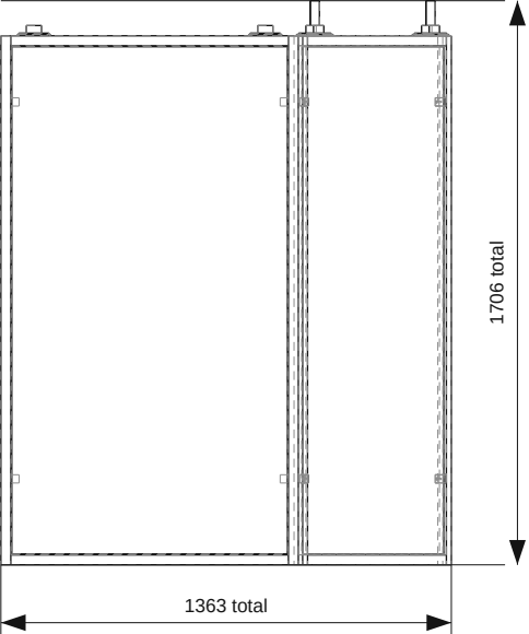
LATERAL (1:25), folhas das pontas de face
