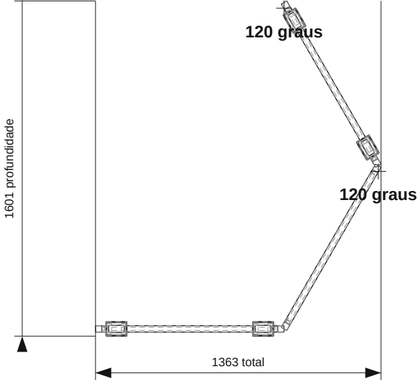
TOPO (1:25), vista de cima
