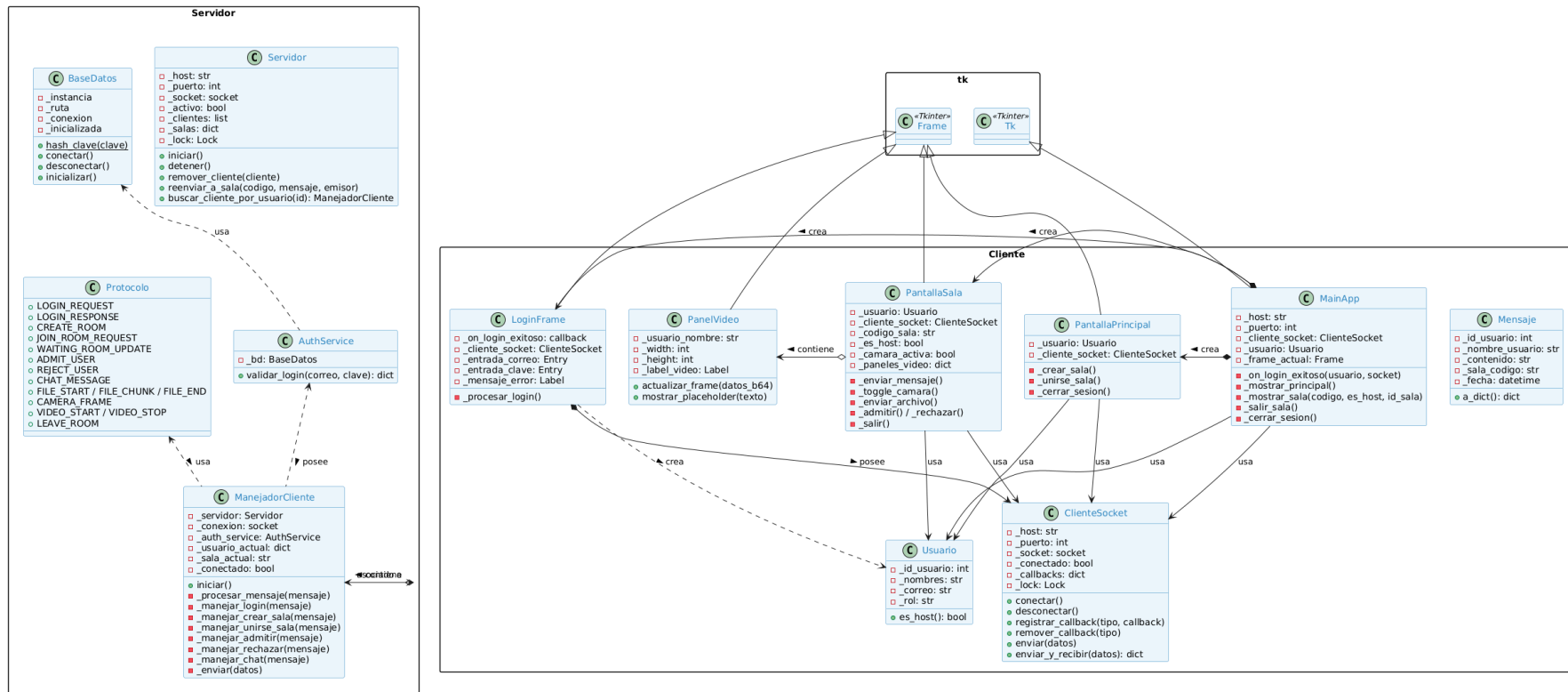
Figura 5: Diagrama de clases del sistema
