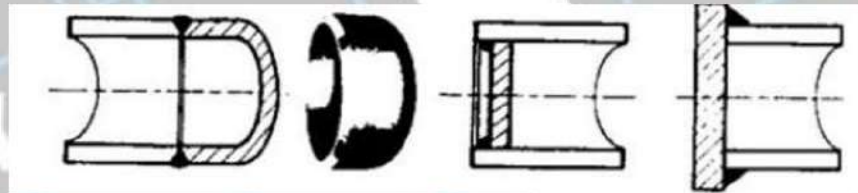
Gambar 2.12 Jenis-jenis cap
