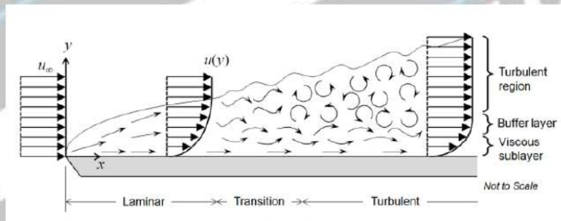
Gambar 2.9 Pusaran arus ( eddy ) yang terjadi pada aliran turbulen Pada teori ini, Danckwert menyatakan asumsi-asumsi berikut:
