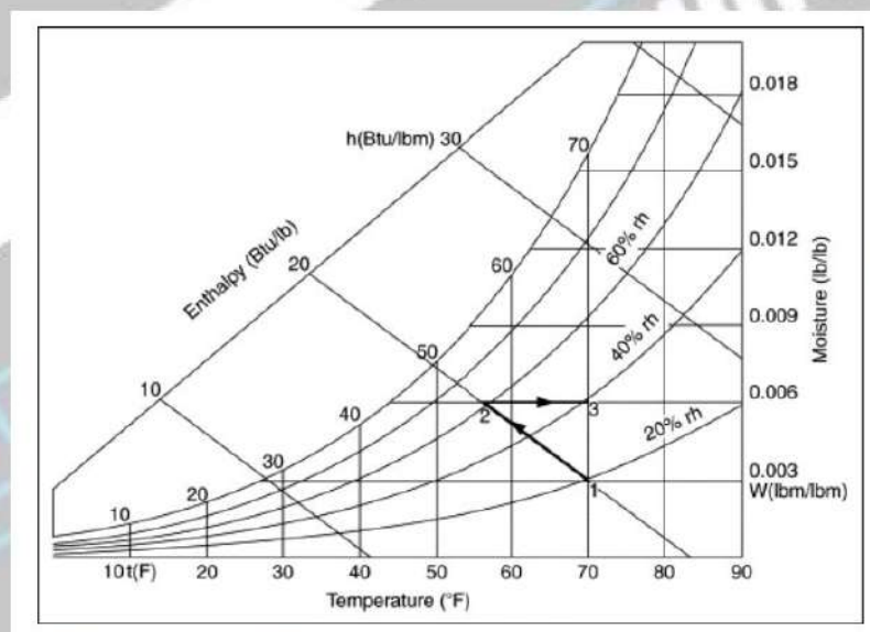
Gambar 2.3 Proses humidifikasi pada psychrometric chart
