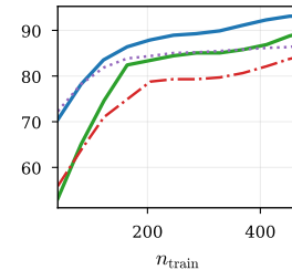
NCI1
