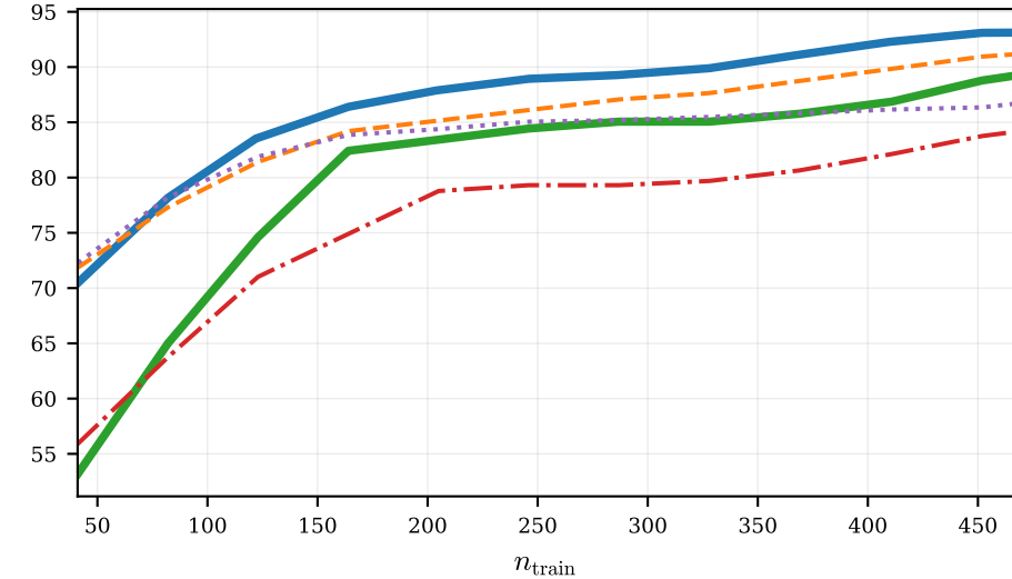
NCI1
