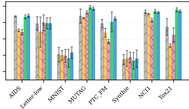
PGExplainer
