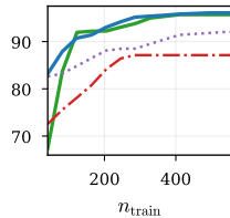
GCN
