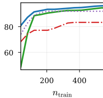
GAT
