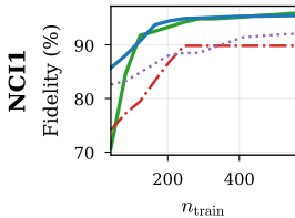
GCN
