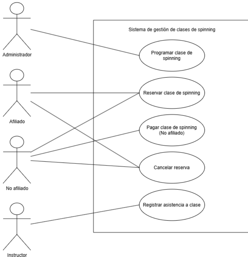
Fig. 6. Diagrama de caso de uso general del sistema.
