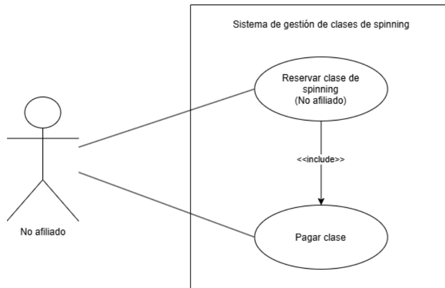
Fig. 2. Diagrama de caso de uso 2: Reservar y pagar clase de spinning.
