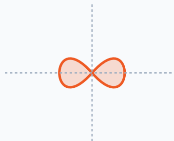
p 오비탈 (방위양자수 l = 1 )
