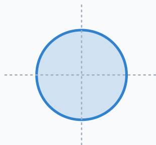
s 오비탈 (방위양자수 l = 0 )
