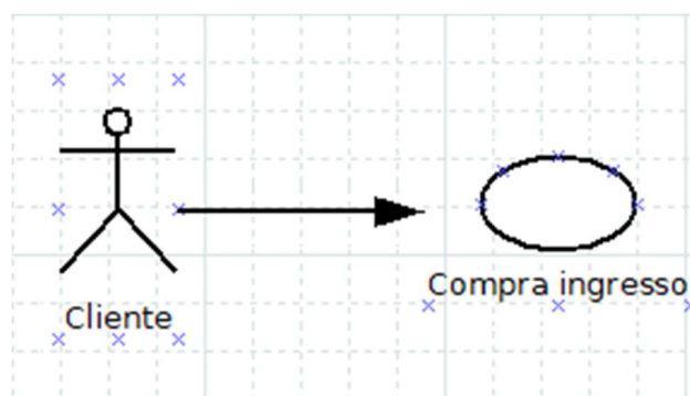
Figura 1 - Relacionamento UML
