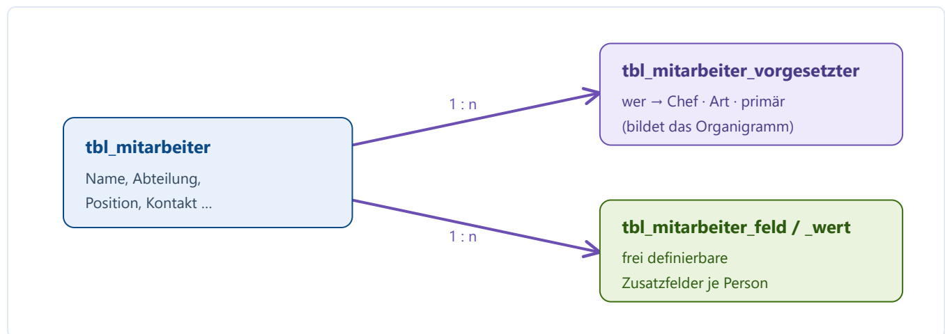
Bild 5 – Ein Mitarbeiter, viele Vorgesetzten-Beziehungen und viele Zusatzfelder.
