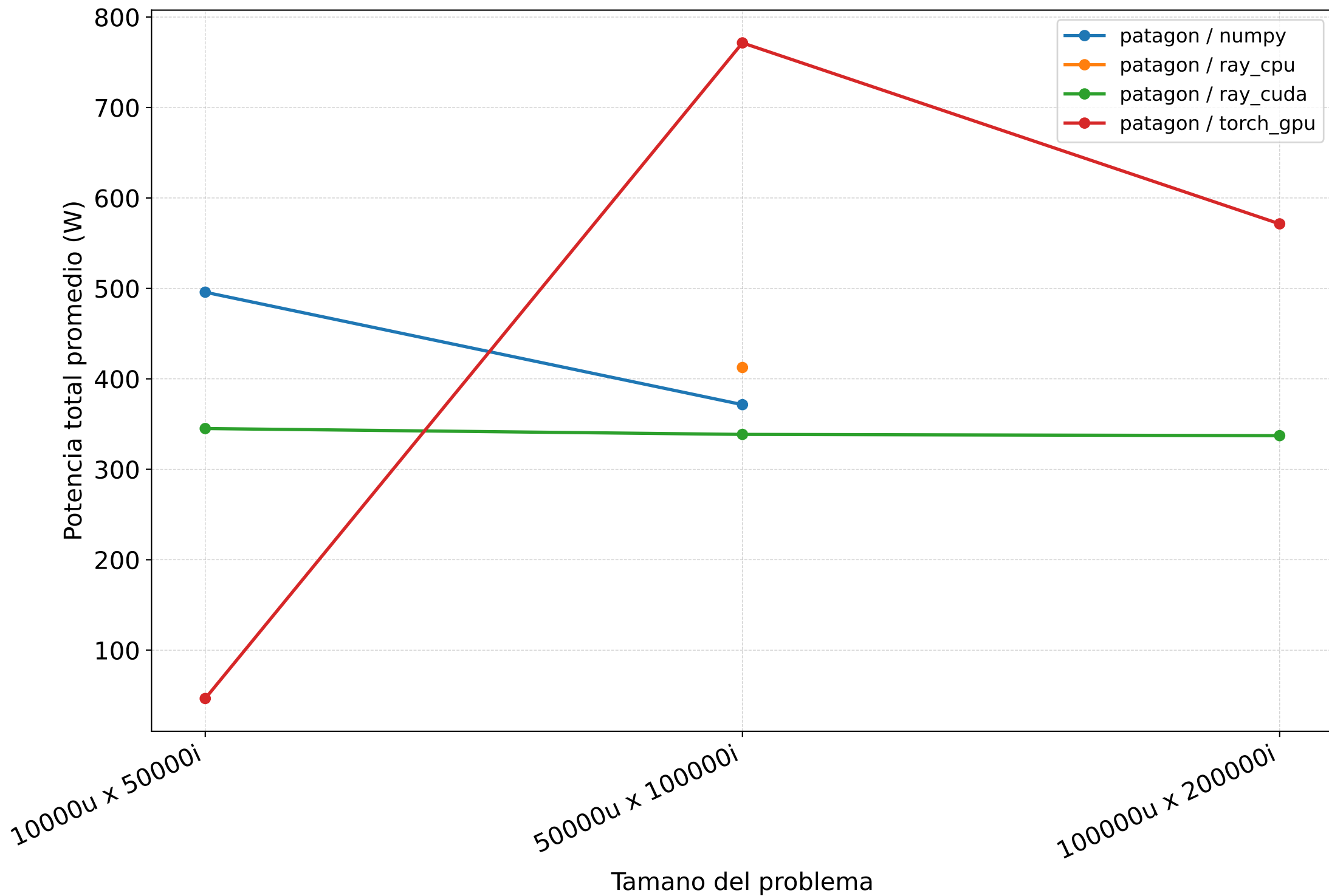
Benchmark recomendador content-based: Potencia total promedio (W)
