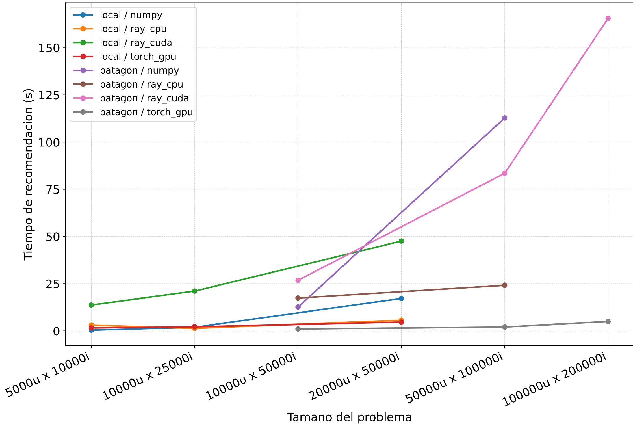
Benchmark recomendador content-based: Tiempo de recomendacion (s)
