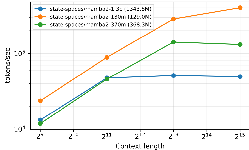
Mamba-2 FP16 Prefill throughput (RTX 5090)
