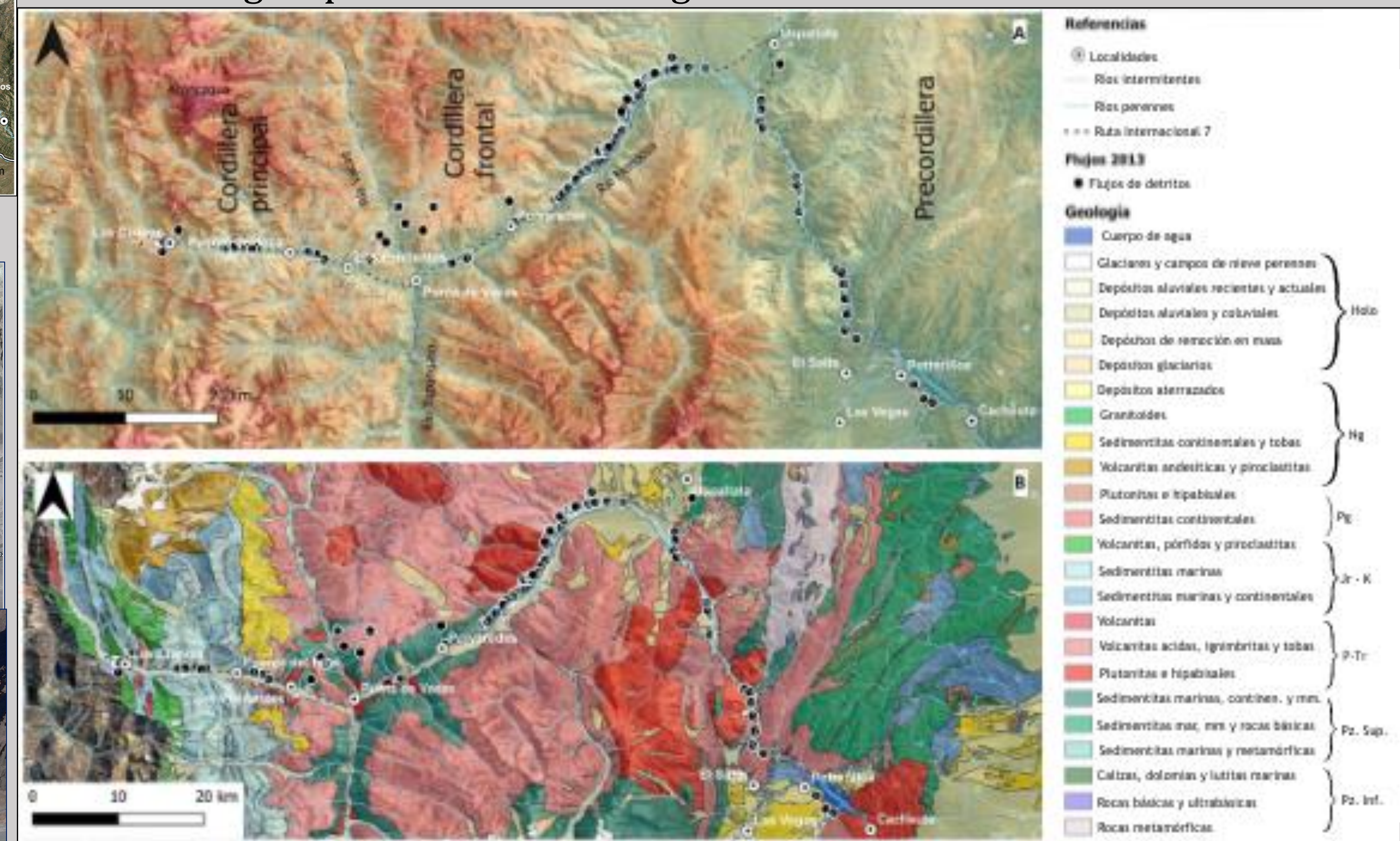
Figura 3. A) Distribución de flujos de detritos ocurridos en enero y febrero de 2013 sobre un modelo de elevación digital. Nótese la distribución de los mismos según las provincias geológicas. B) Mapa geológico regional obtenido del SEGEMAR donde se observa la mayor participación de flujos de detritos relacionados con las rocas del Grupo Choiyoi.
