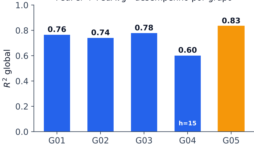
FedPer + FedAvg - desempenho por grupo
