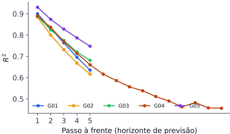
R 2 por passo de previsão - FedPer+FedAvg
