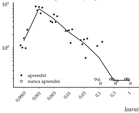
gradient disparity
