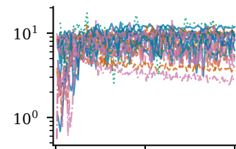
mcoh/global
