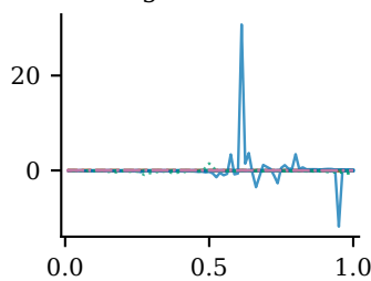
gwa/value
