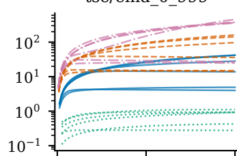
gsnr/mean
