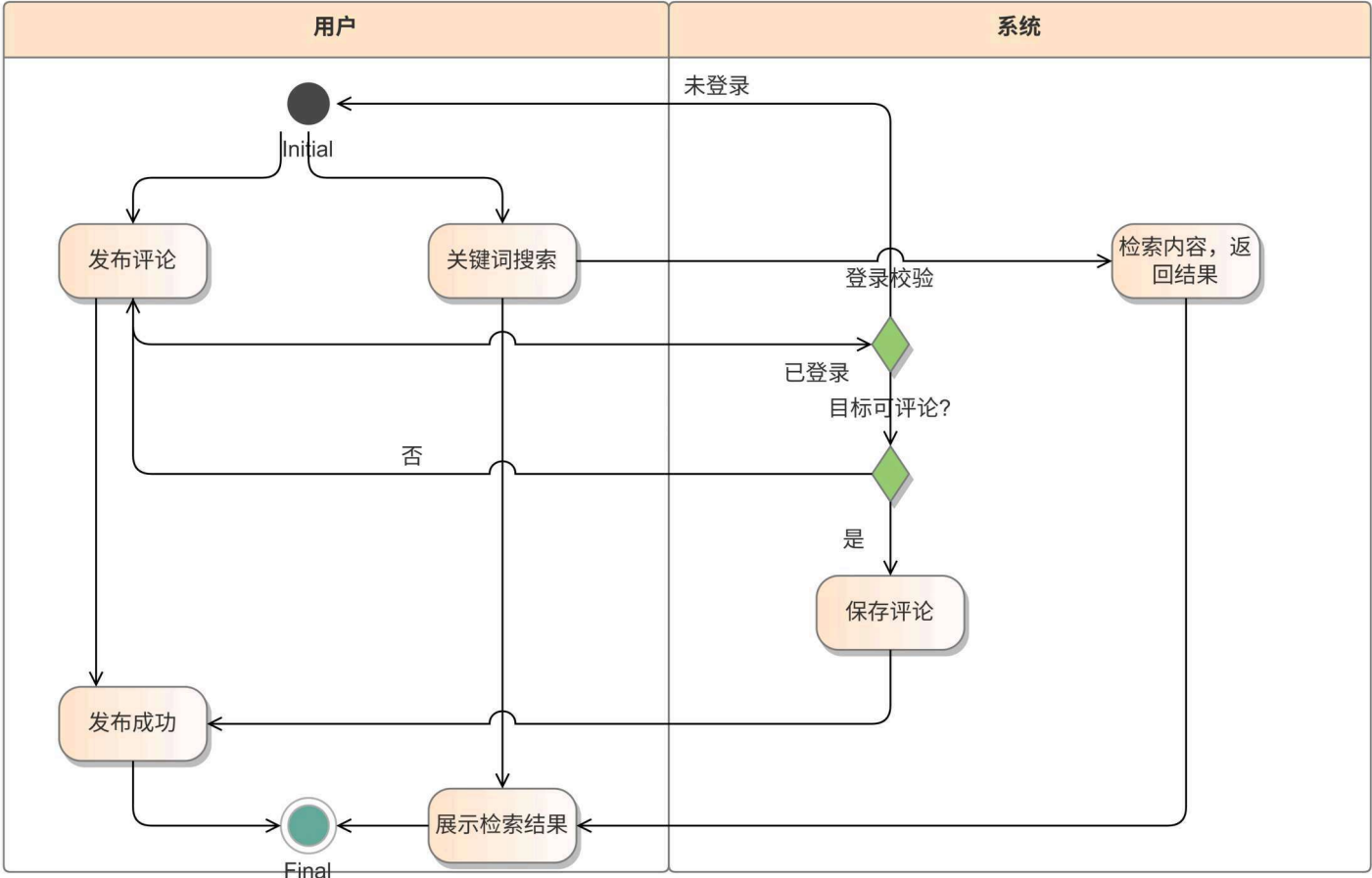
2.6活动图.png
