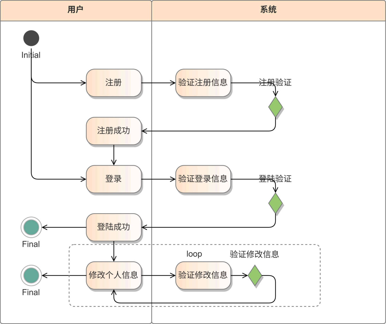
2.1活动图.png
