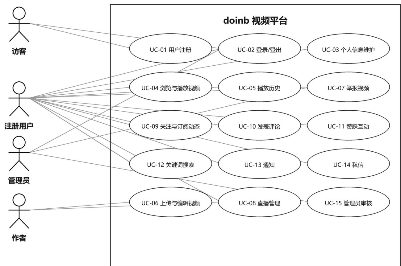
usecase.png
