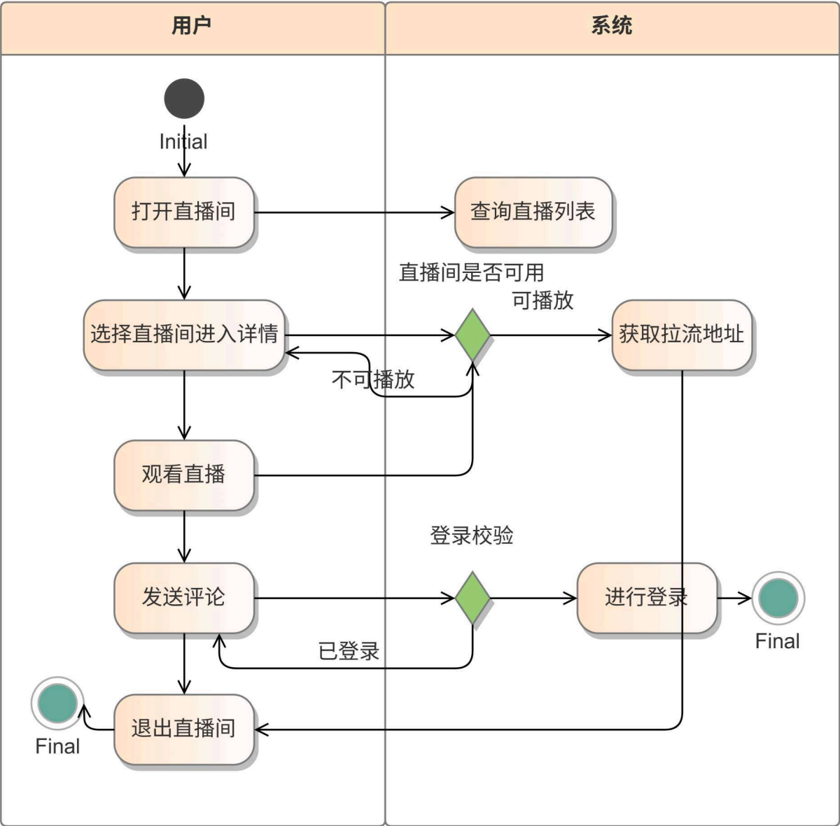
2.3活动图.png
