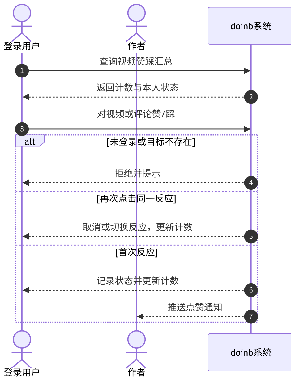
图 3-13 UC-11 赞踩互动系统顺序图
