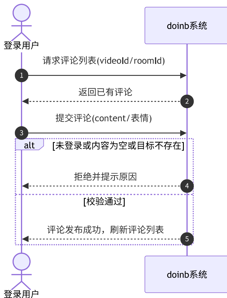
图 3-12 UC-10 发表评论系统顺序图
