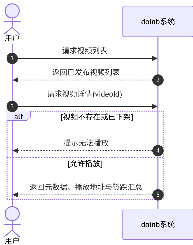
图 3-6 UC-04 浏览与播放视频系统顺序图
