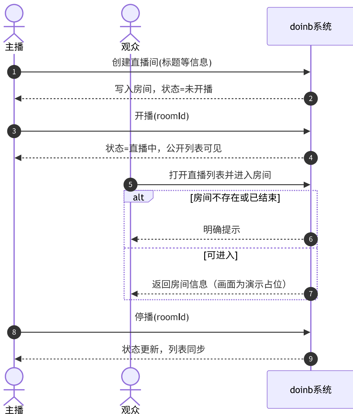
图 3-10 UC-08 直播管理系统顺序图
