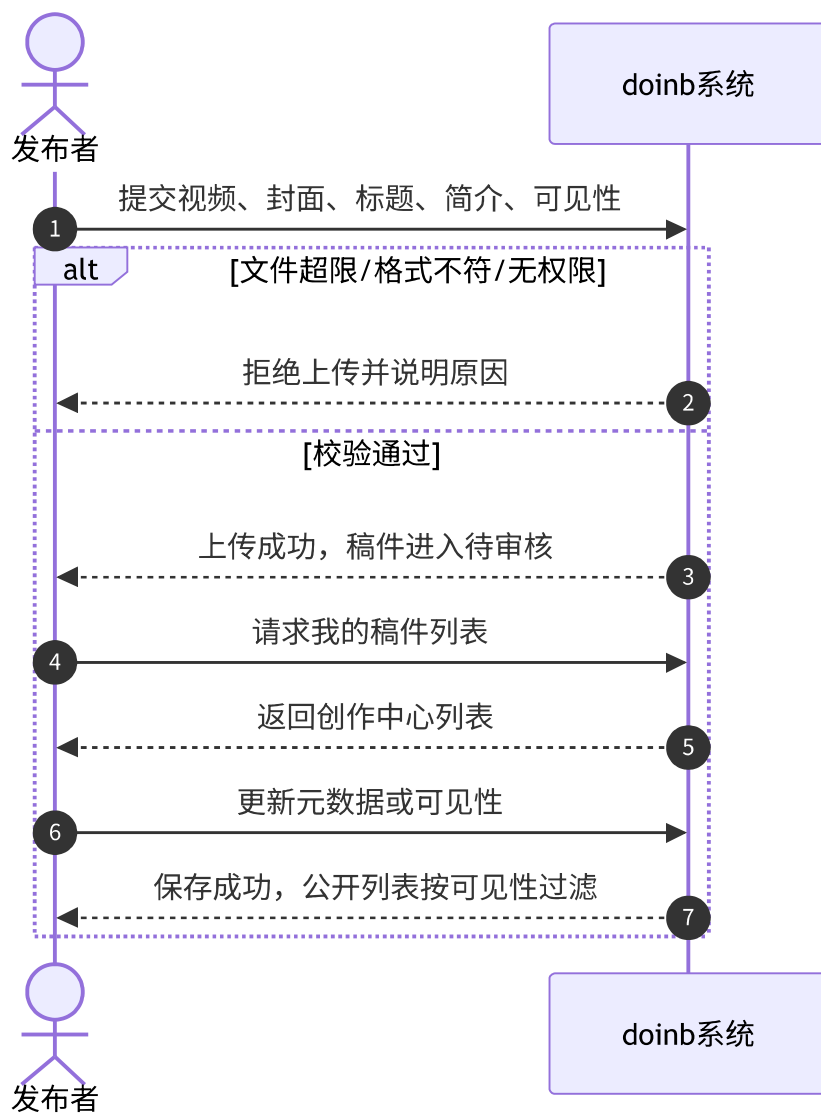
图 3-8 UC-06 上传与编辑视频系统顺序图
