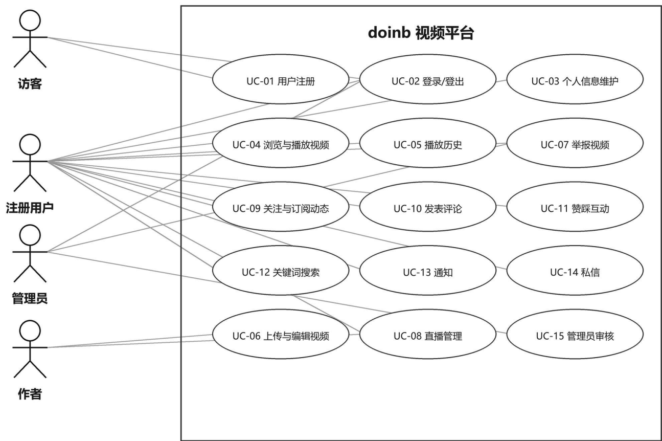
图 3-1 系统用例图
