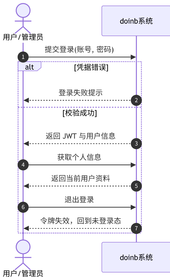
图 3-4 UC-02 用户登录/登出系统顺序图
