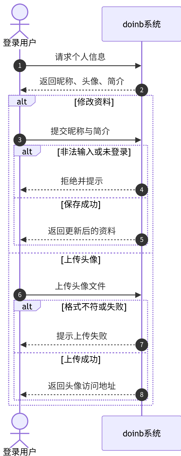
图 3-5 UC-03 个人信息维护系统顺序图
