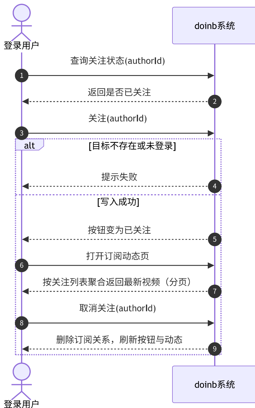
图 3-11 UC-09 关注与订阅动态系统顺序图
