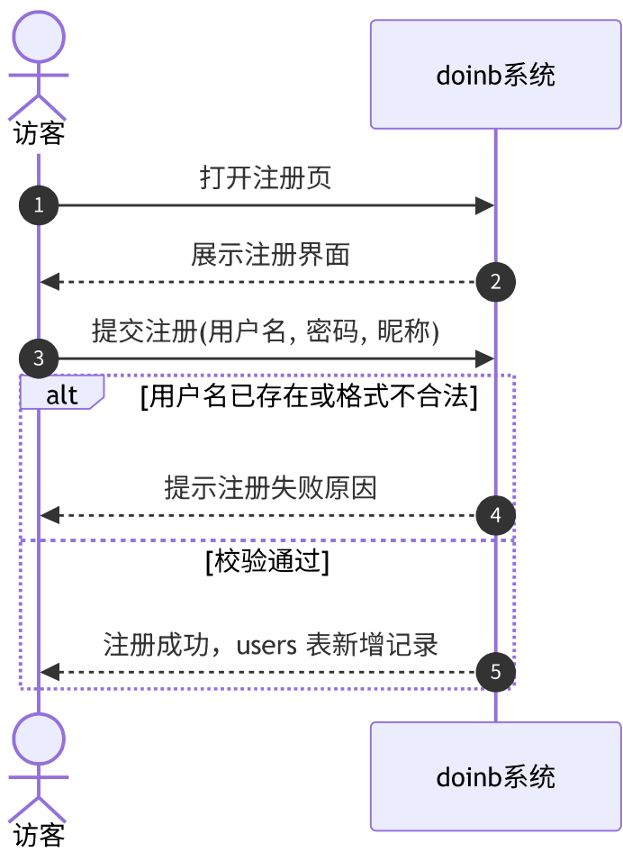
图 3-3 UC-01 用户注册系统顺序图
