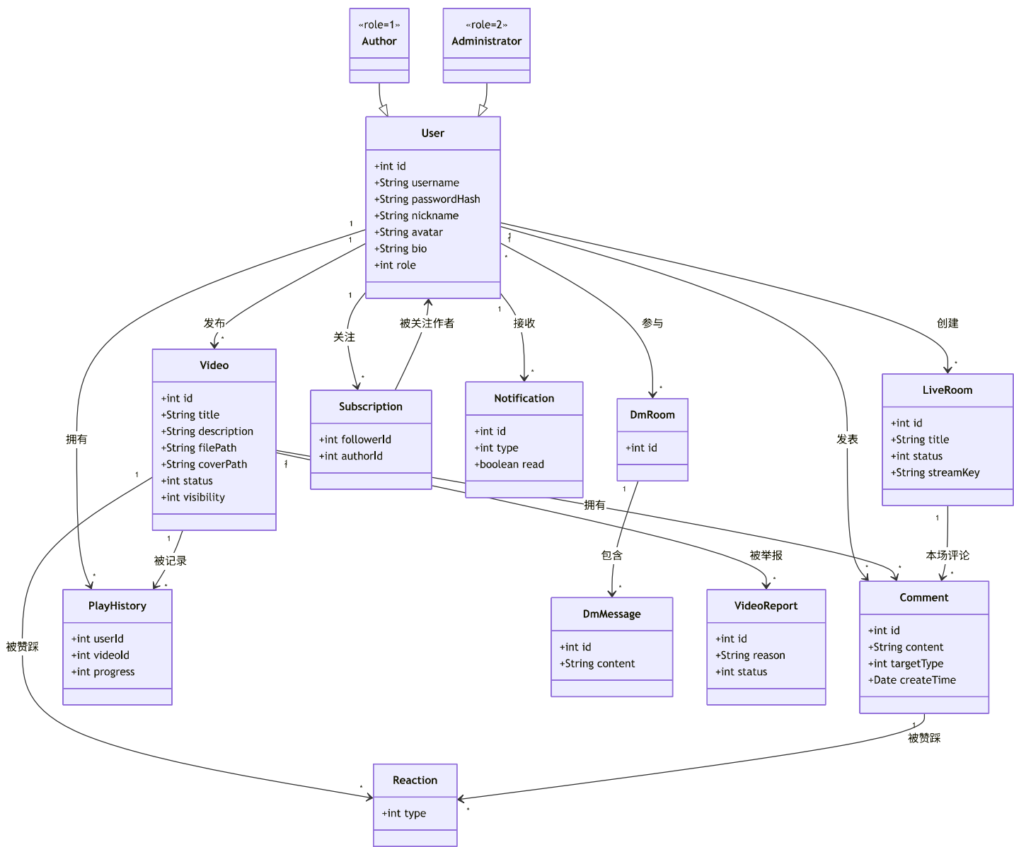
图 3-2 领域概念类图
