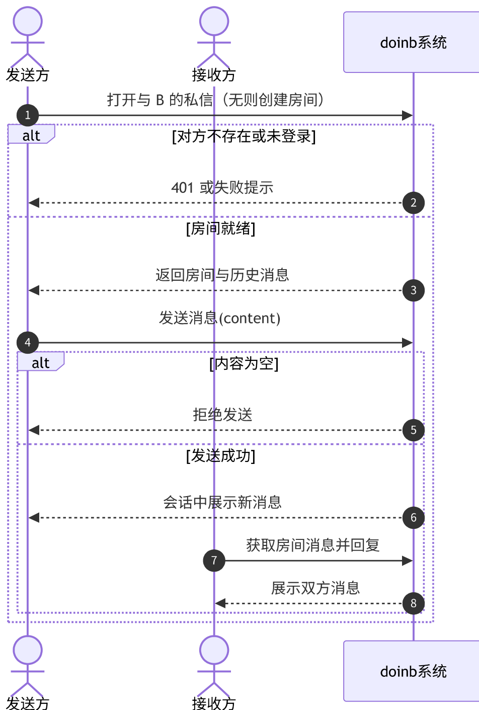
图 3-16 UC-14 私信系统顺序图
