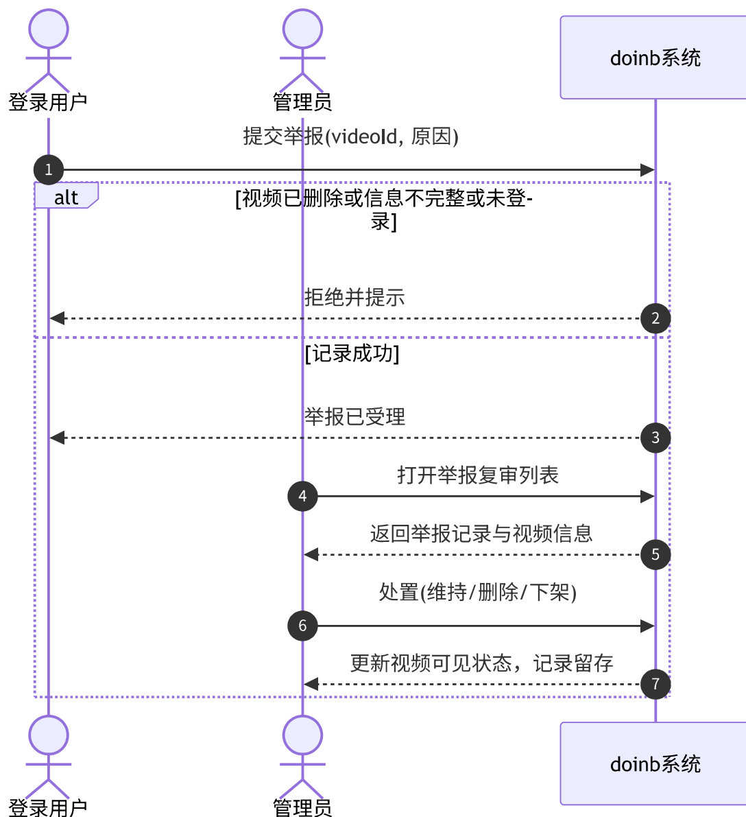
图 3-9 UC-07 举报视频系统顺序图
