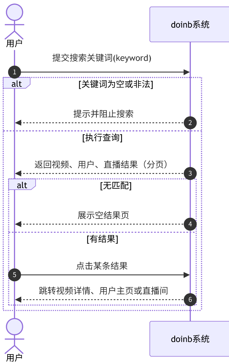
图 3-14 UC-12 关键词搜索系统顺序图
