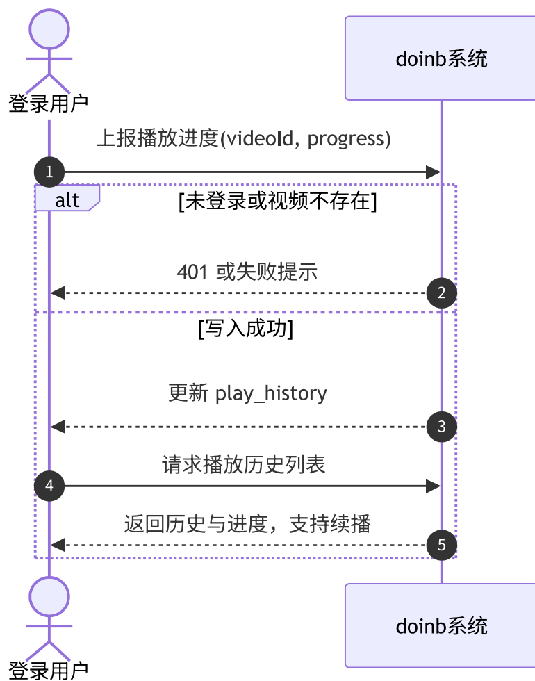
图 3-7 UC-05 播放历史系统顺序图
