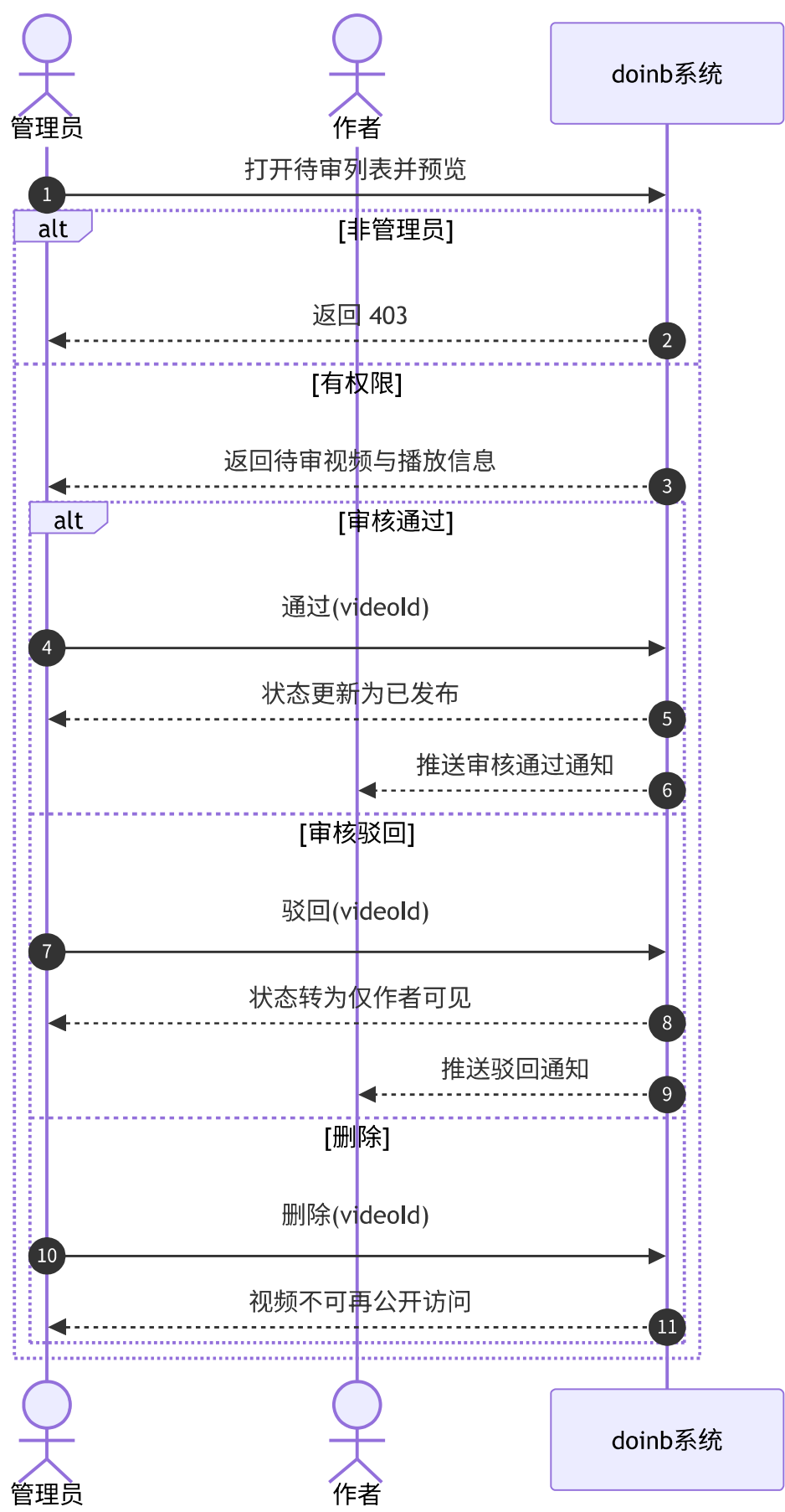
图 3-17 UC-15 管理员审核系统顺序图
