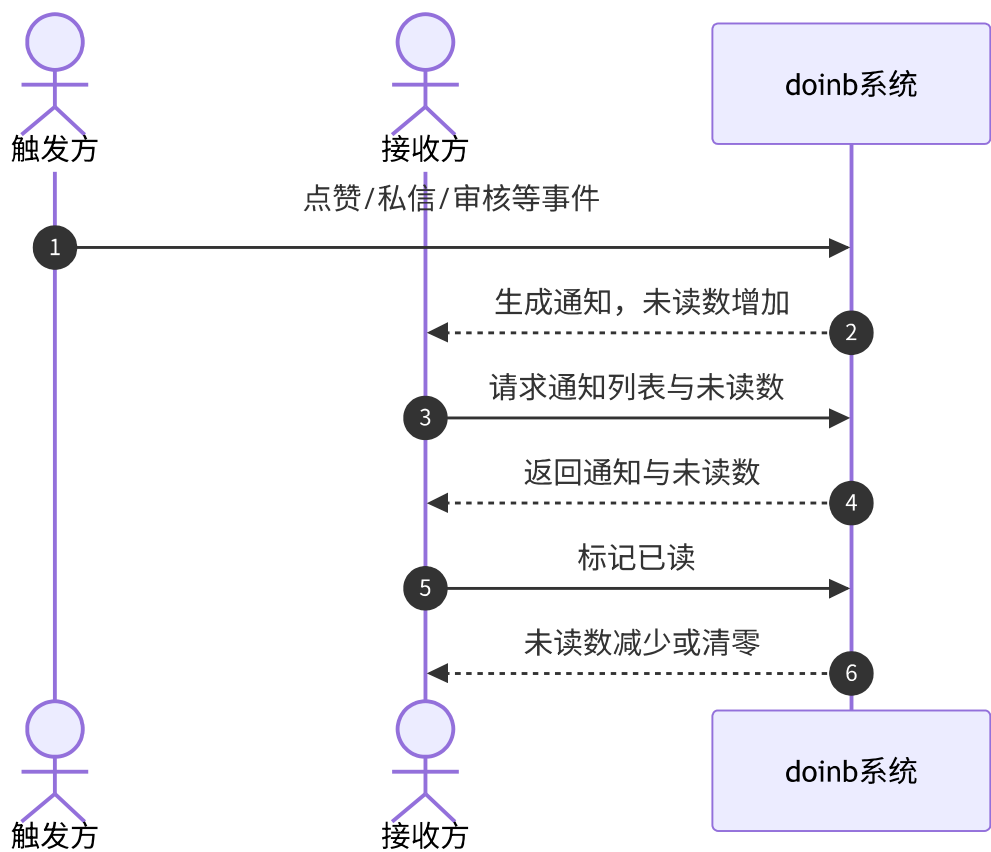
图 3-15 UC-13 通知系统顺序图
