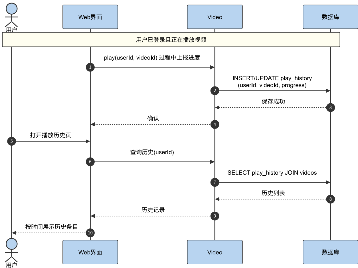
记录播放历史的顺序图：
