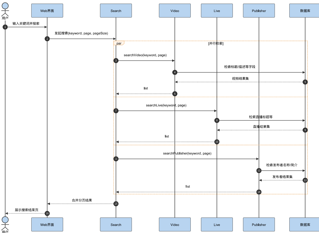
关键词搜索的顺序图：
