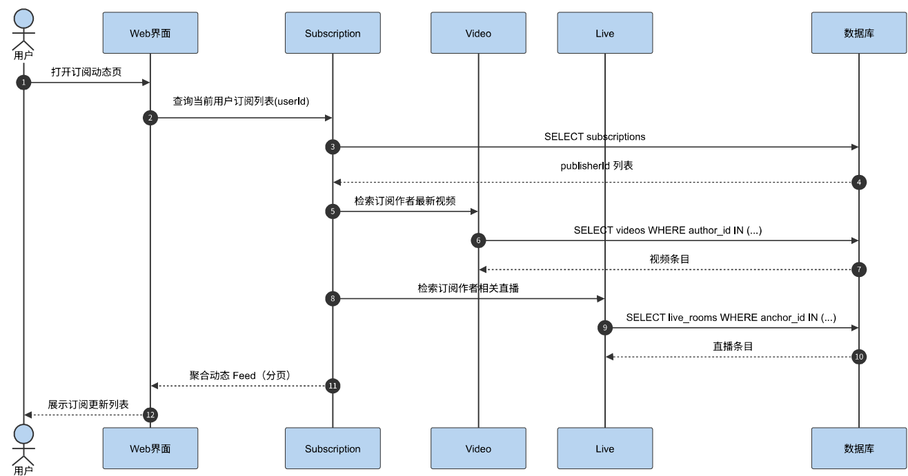
查看订阅动态的顺序图：
