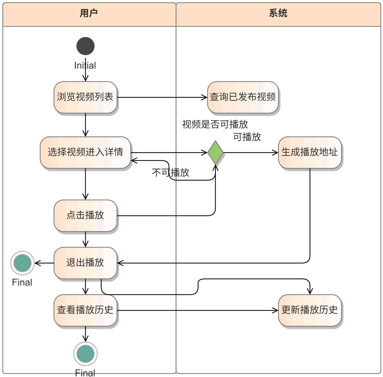
图 2-5 视频播放子系统活动图
