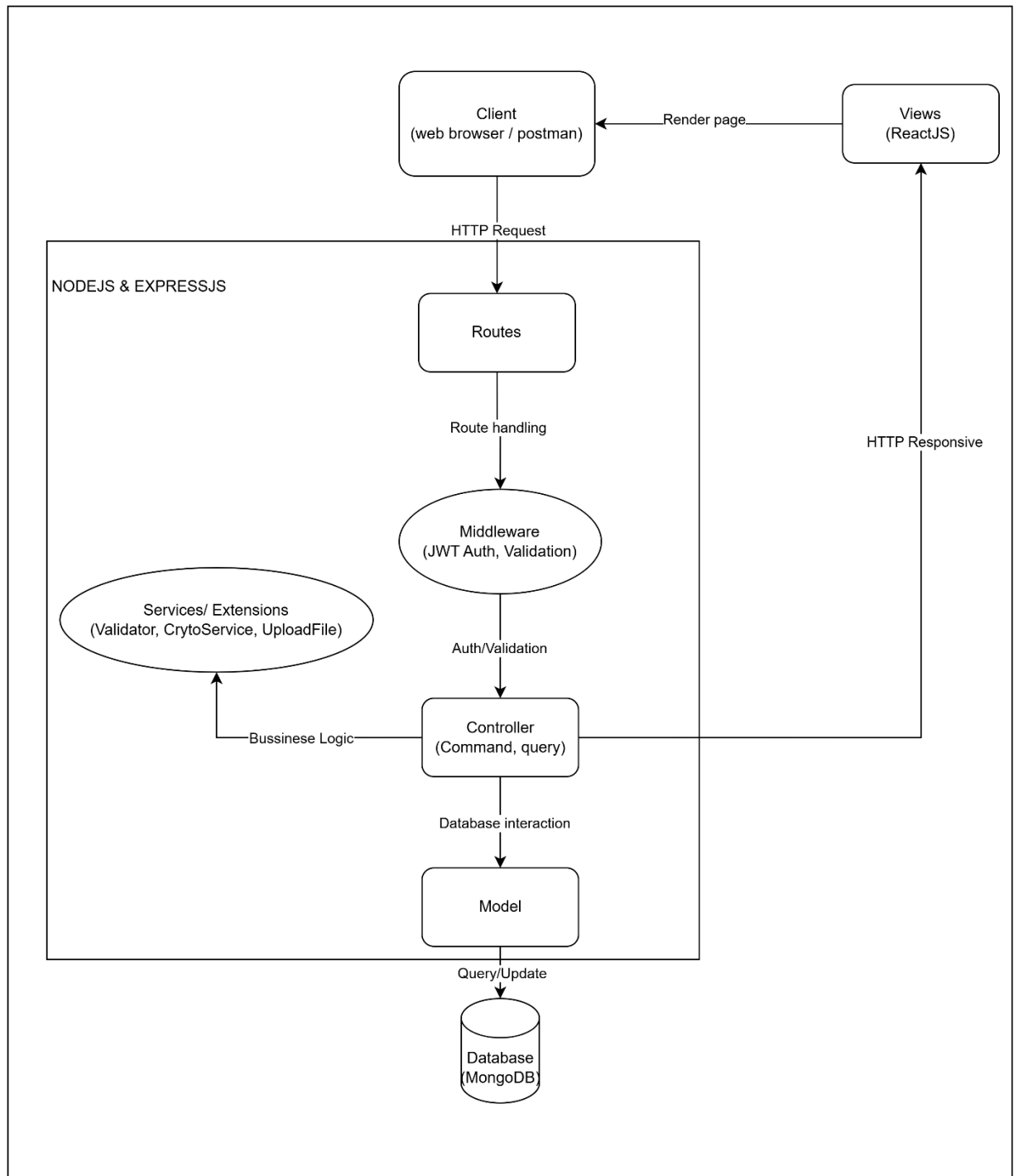
Hình 2.8 Kiến trúc hệ thống
