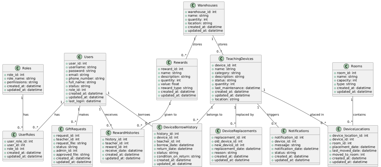
Hình 2.3 Sơ đồ lớp
