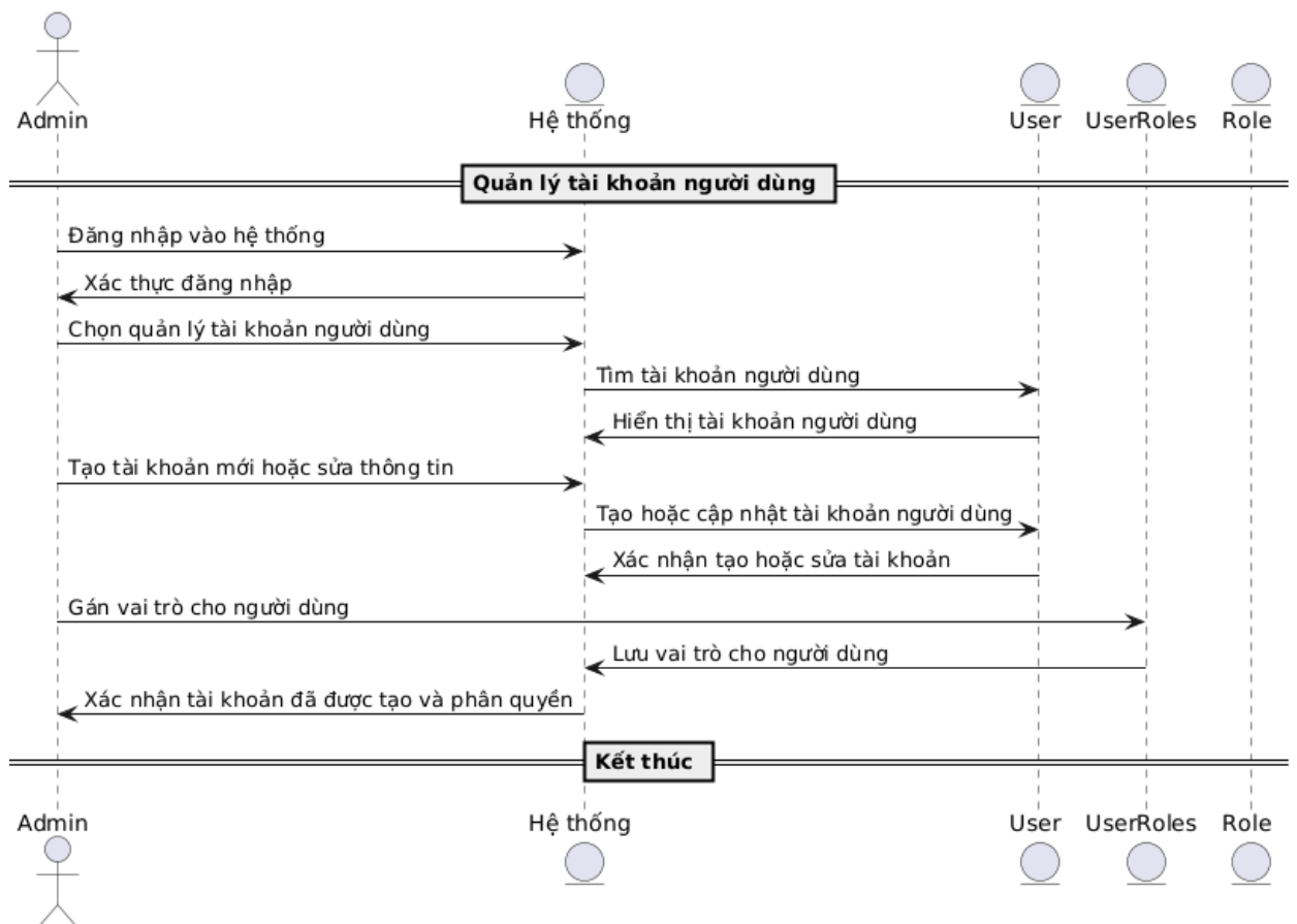
Hình 2.4 Sơ đồ tuần tự quản lý người dùng
