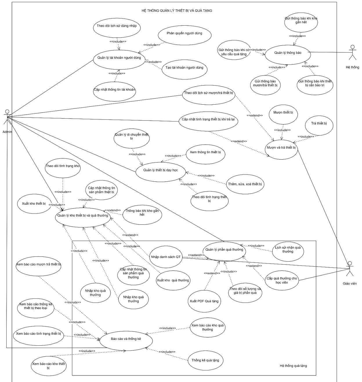
Hình 2.2 Sơ đồ use case
