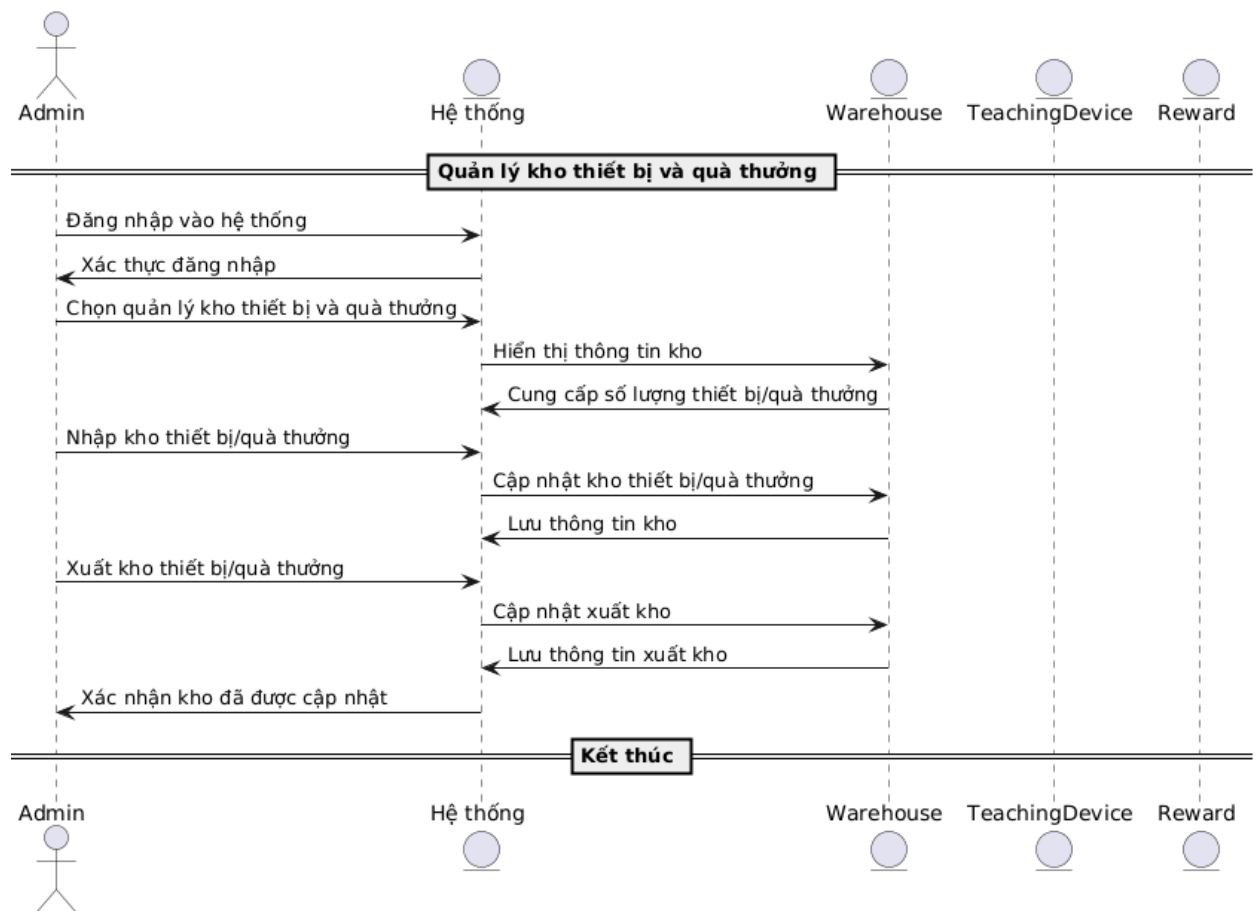
Hình 2.6 Sơ đồ tuần tự quản lý kho thiết bị và quà tặng
