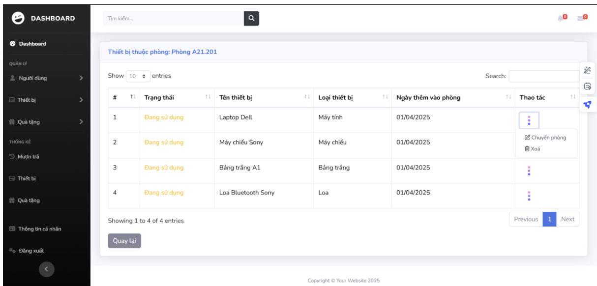
Hình 2.22 Giao diện xem thiết bị trong phòng
