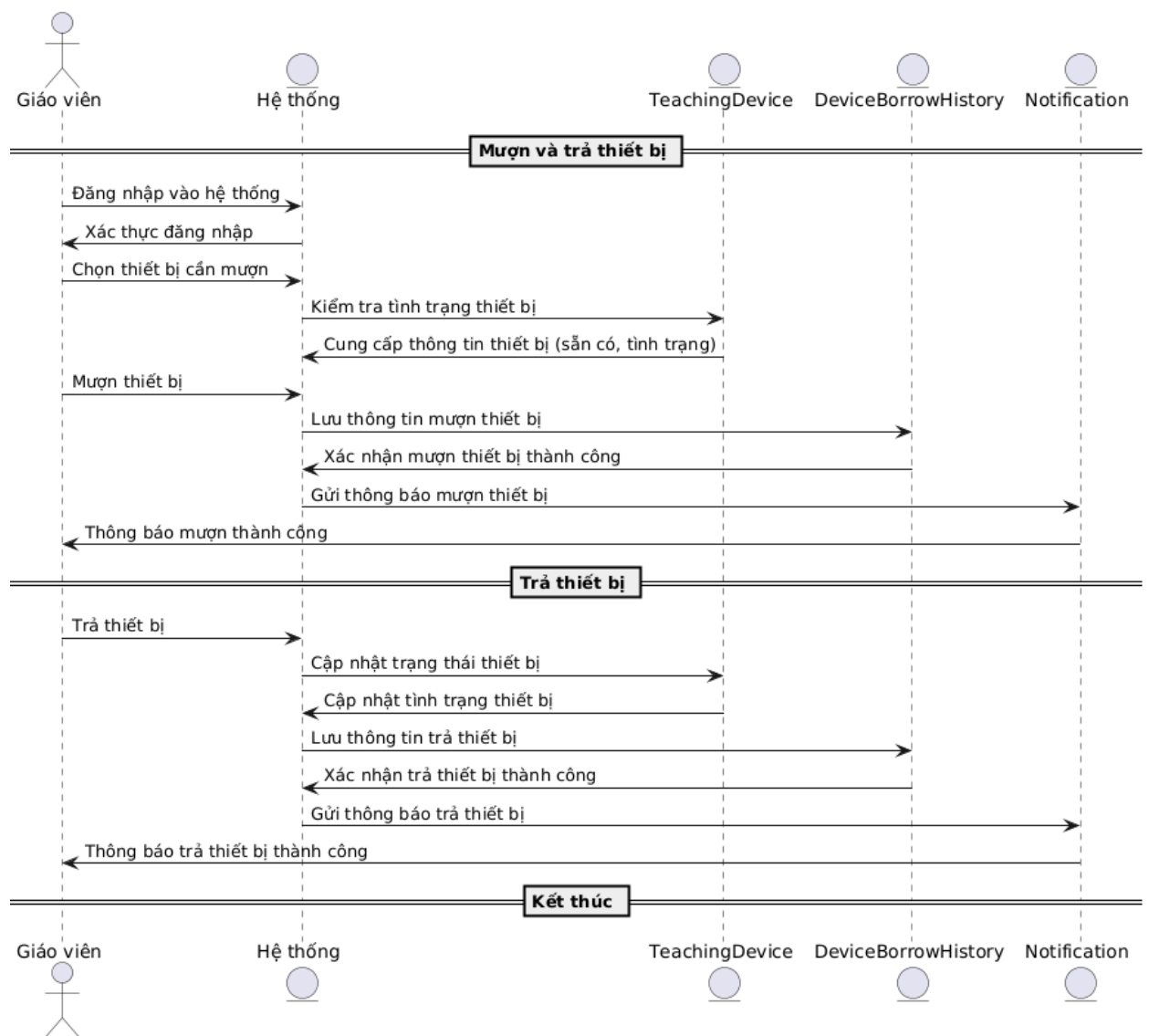
Hình 2.5 Sơ đồ tuần tự mượn/trả thiết bị
