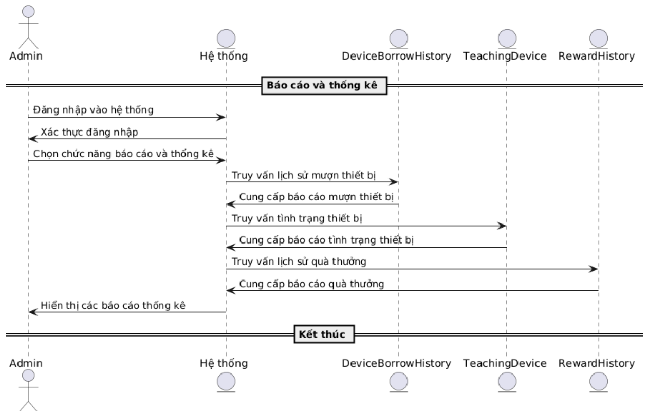
Hình 2.7 Sơ đồ tuần tự báo cáo và thống kê
