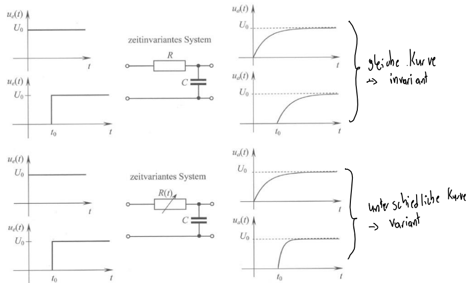
Bild 9.5 Zeitinvariantes und zeitvariantes System
