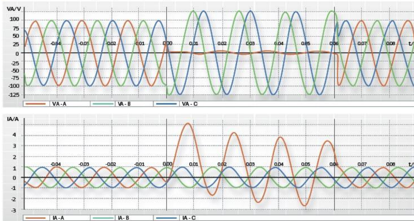
Figure 4: Aufzeichnung eines Einphasen-Erdschlussfehlers
