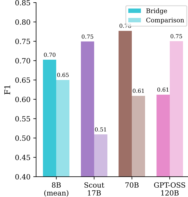
(b) Bridge vs. Comparison F1
