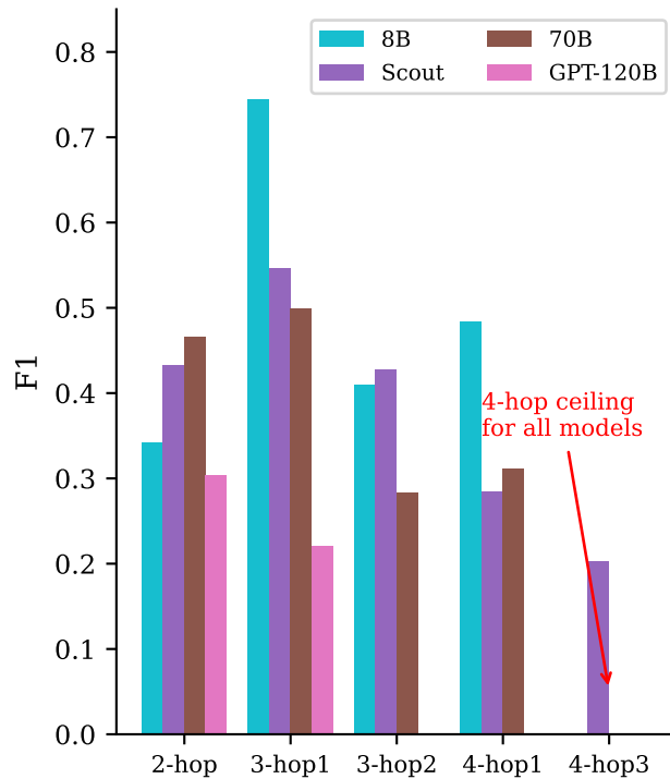
(b) F1 by Hop Count
