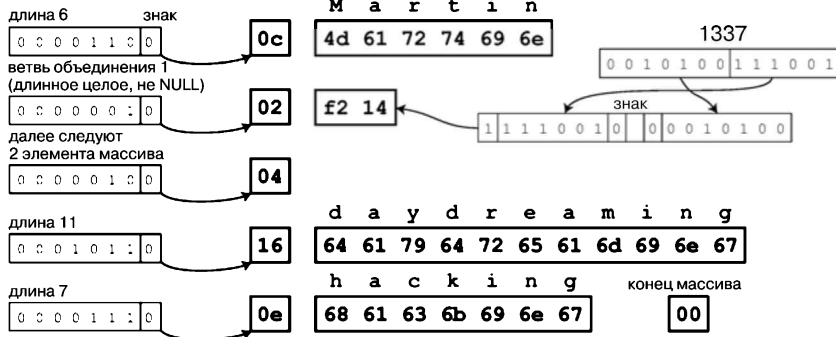
Рис. 4.5. Наш пример записи, закодированный с помощью Avro
