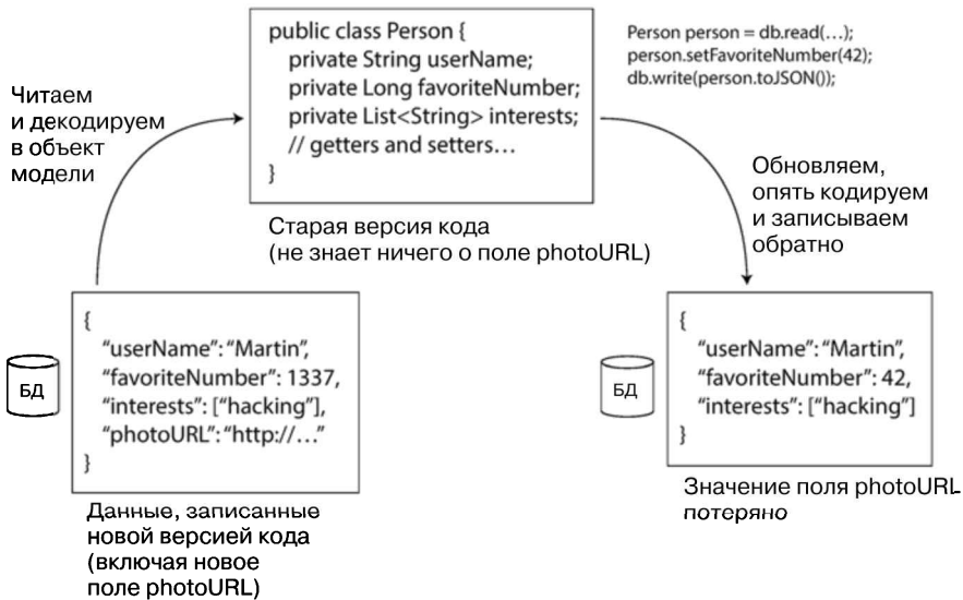
Рис. 4.7. Если не быть аккуратными, то можно потерять данные при обновлении старой версией приложения данных, ранее записанных более новой его версией
