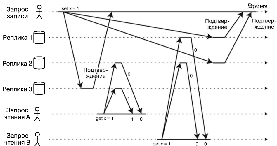
Рис. 9.6. Несмотря на строгий кворум, операции выполняются нелинейаризуемо
