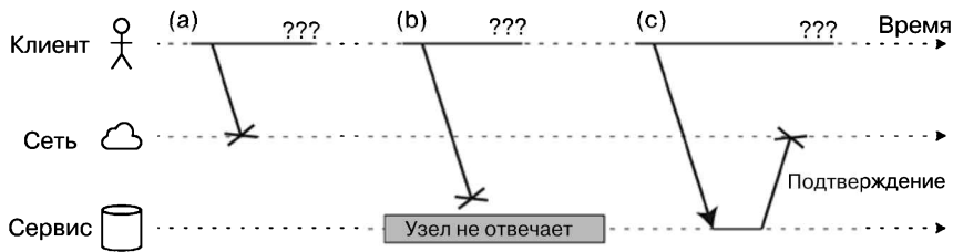
Рис. 8.1. В случае отправки запроса и неполучения ответа невозможно определить: а) был ли потерян запрос; б) работает ли удаленный узел; в) не был ли потерян ответ
