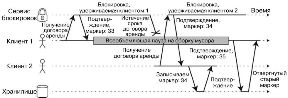
Рис. 8.5. Безопасный доступ к хранилищу благодаря тому, что операции записи разрешаются только в порядке возрастания ограждающих маркеров
