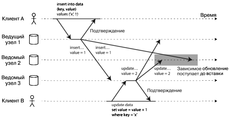
Рис. 5.9. При репликации с несколькими ведущими узлами информация об операциях записи может поступать в некоторые реплики в неправильном порядке
