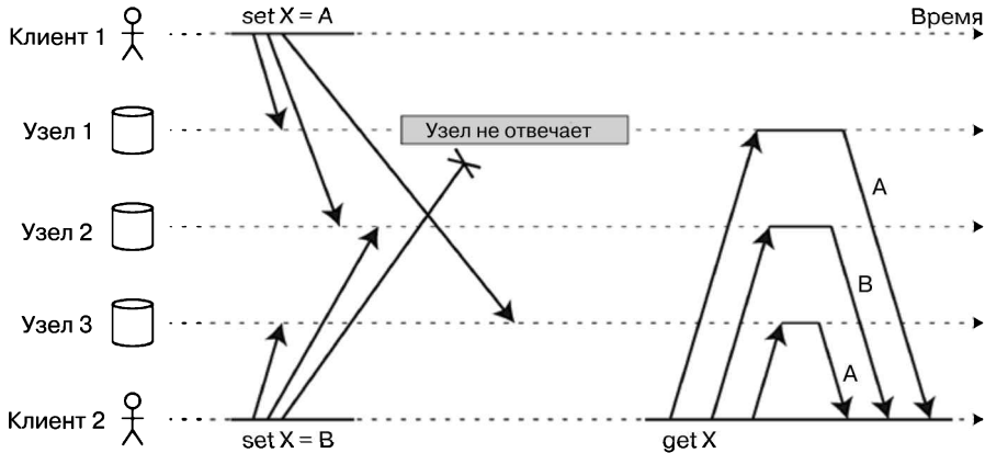
Рис. 5.12. Конкурентные операции записи в Дупато-подобном складе данных: четко определенный порядок отсутствует
