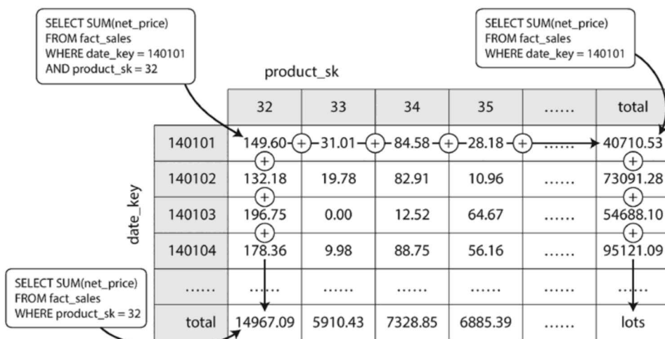
Рис. 3.12. Два измерения куба данных, агрегирующих данные путем суммирования
