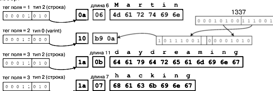
Рис. 4.4. Наш пример записи, закодированный с помощью Protocol Buffers
