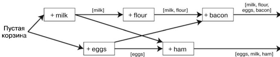
Рис. 5.14. Граф причинно-следственных зависимостей с рис. 5.13
