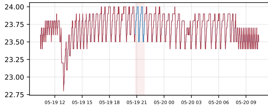
dropout (medium)
