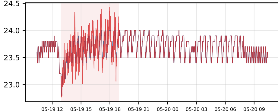
noise (medium)
