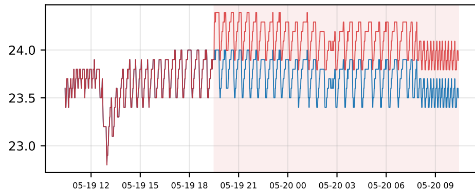
dropout (medium)
