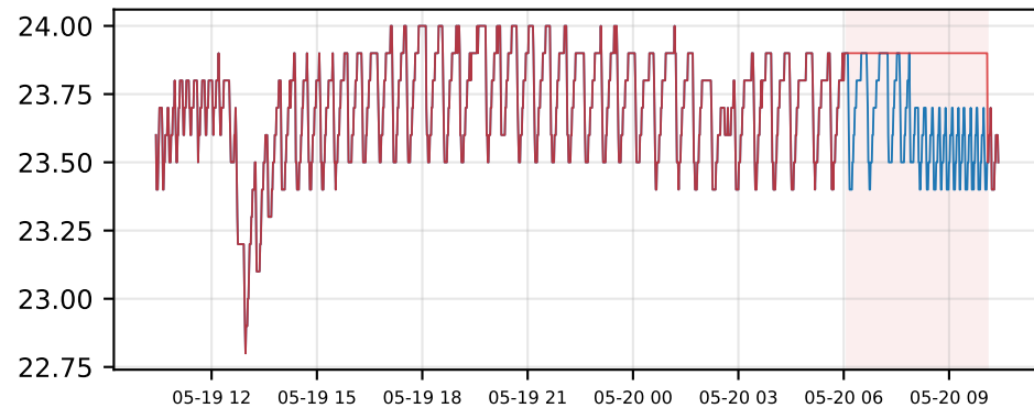
bias (medium)
