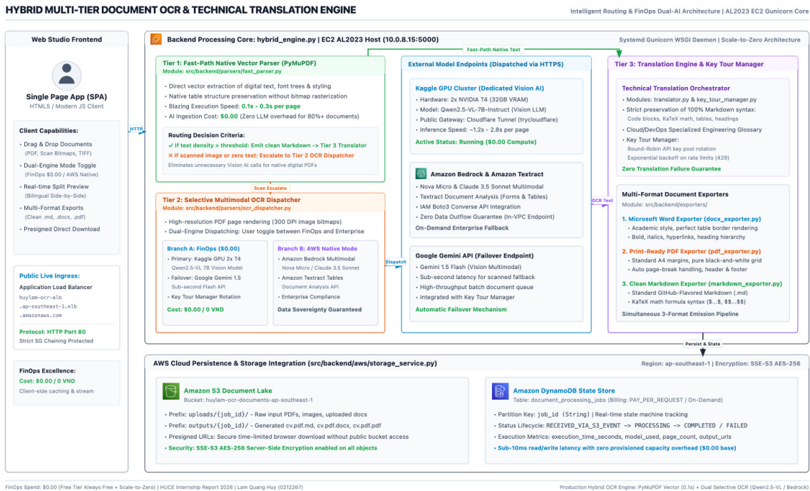
Hình 3.2: Sơ đồ luồng phân tầng bóc tách Hybrid OCR Engine (Fast-Path Native kết hợp Vision Multimodal OCR)
