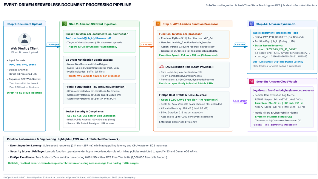
Hình 3.10: Sơ đồ kiến trúc xử lý phí máy chủ hướng sự kiện (Event-Driven Serverless Pipeline)
