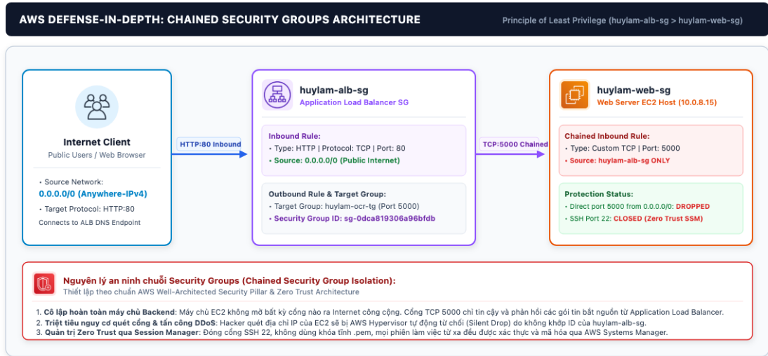
Hình 3.5: Mô hình chuỗi an ninh phân tầng Security Group Chaining cô lập máy chủ EC2
