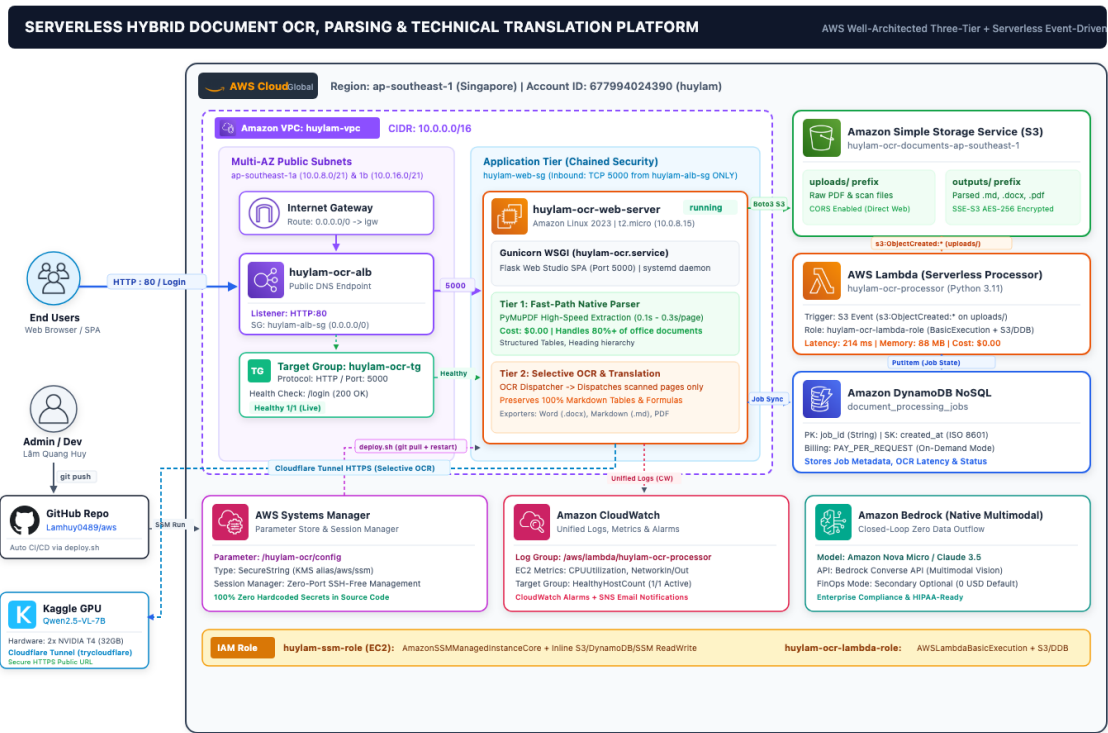
Hình 3.1: Sơ đồ kiến trúc tổng thể hệ thống Serverless Hybrid Document OCR trên nền tảng đám mây AWS
