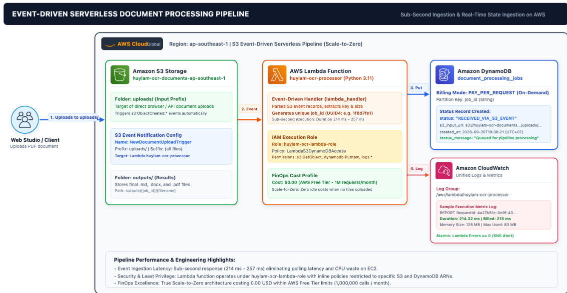
Hình 3.10: Sơ đồ kiến trúc xử lý phí máy chủ hướng sự kiện (Event-Driven Serverless Pipeline)
