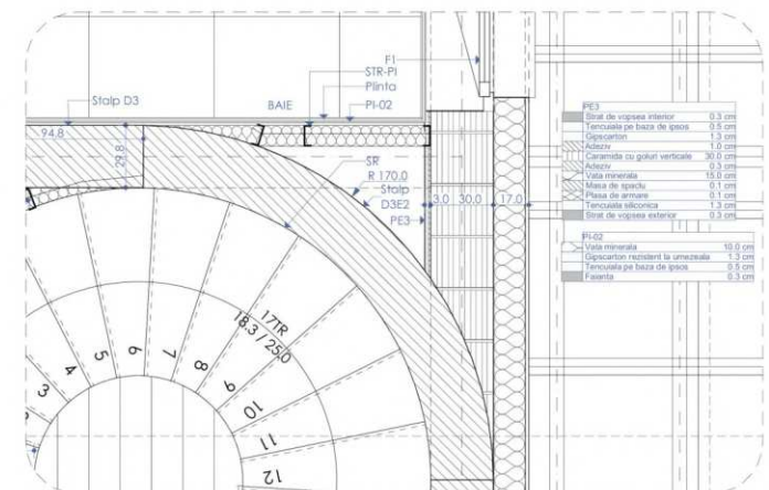
D.E.02 DETALIU 1:10
