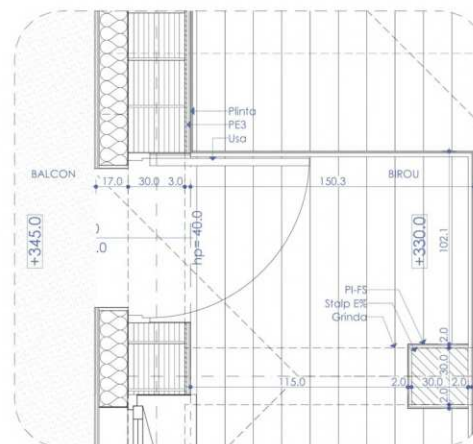
D.E.01 DETALIU 1:10
