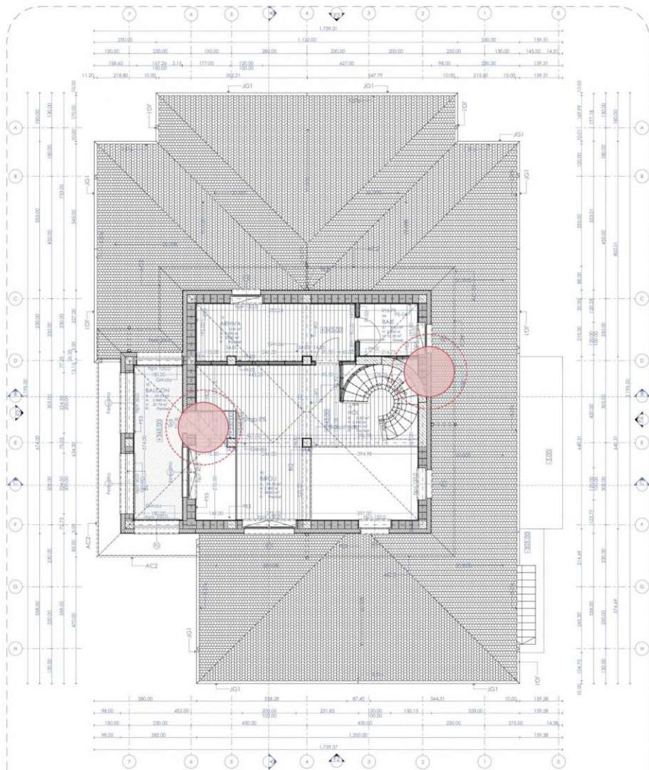
PLAN ETAJ 1:50
