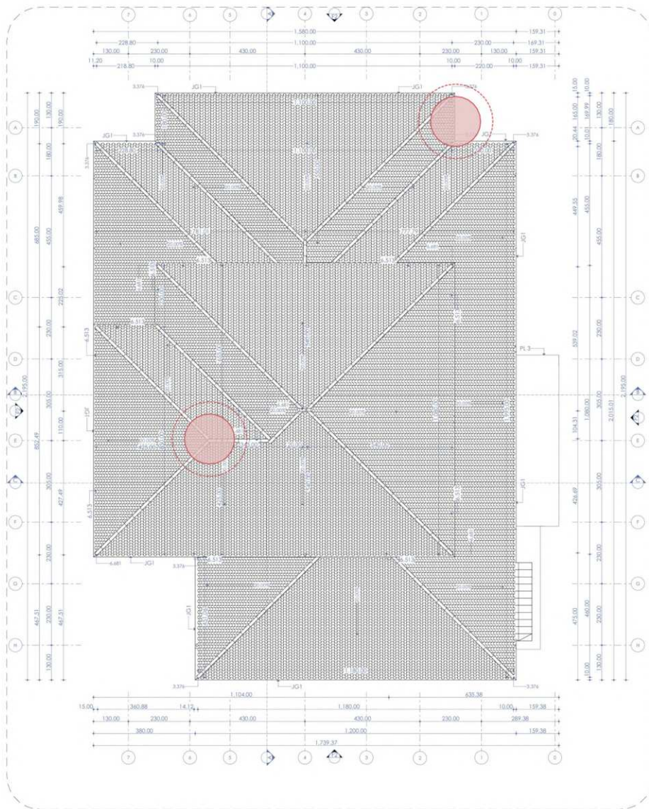
PLAN ACOPERIS 1:50
