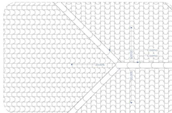
D.A.01 DETALIU 1:10
