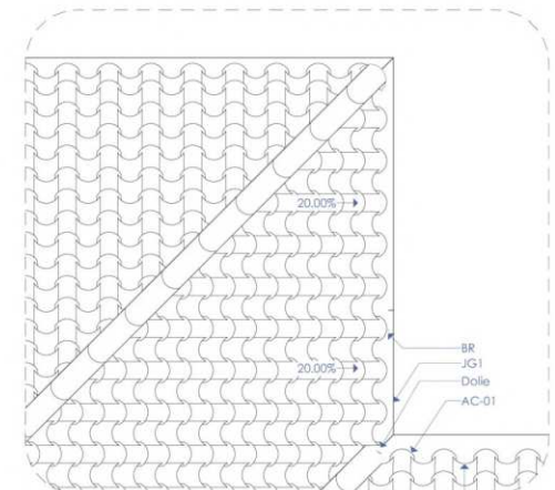
D.A.02 DETALIU 1:10
