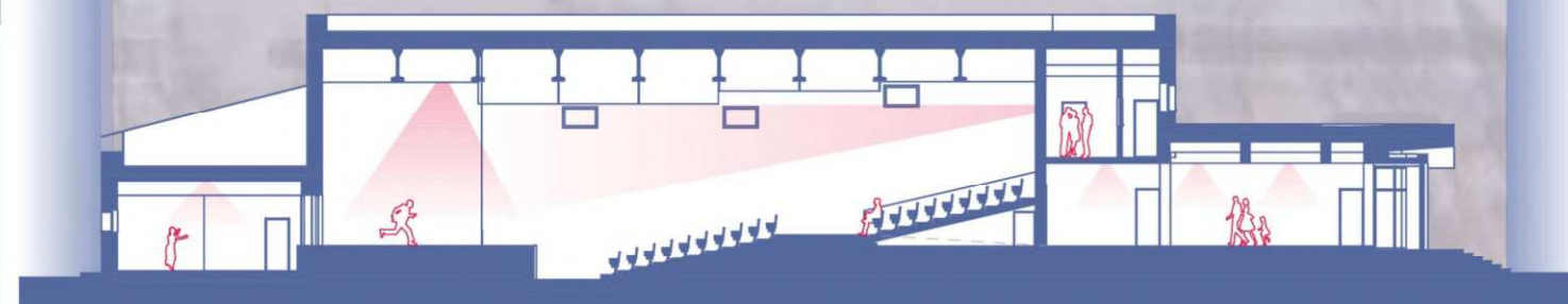
SECTIUNE A-A 1:150
