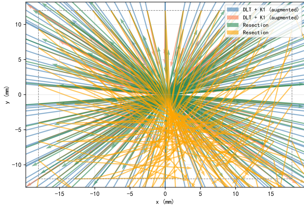
畸变矢量场 (放大5000倍)
