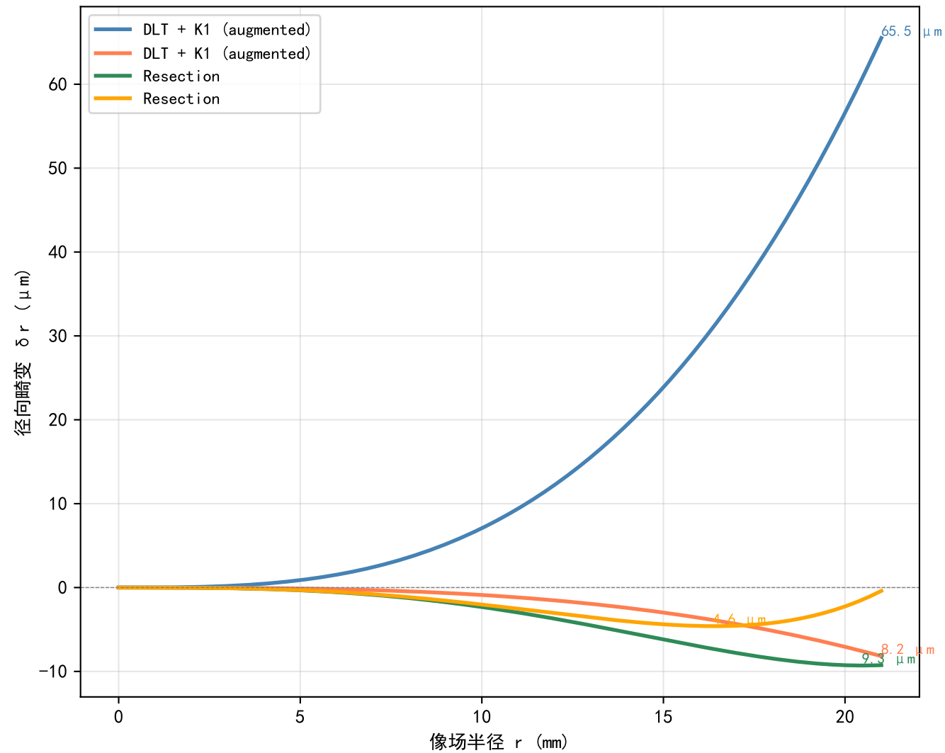
径向畸变曲线
