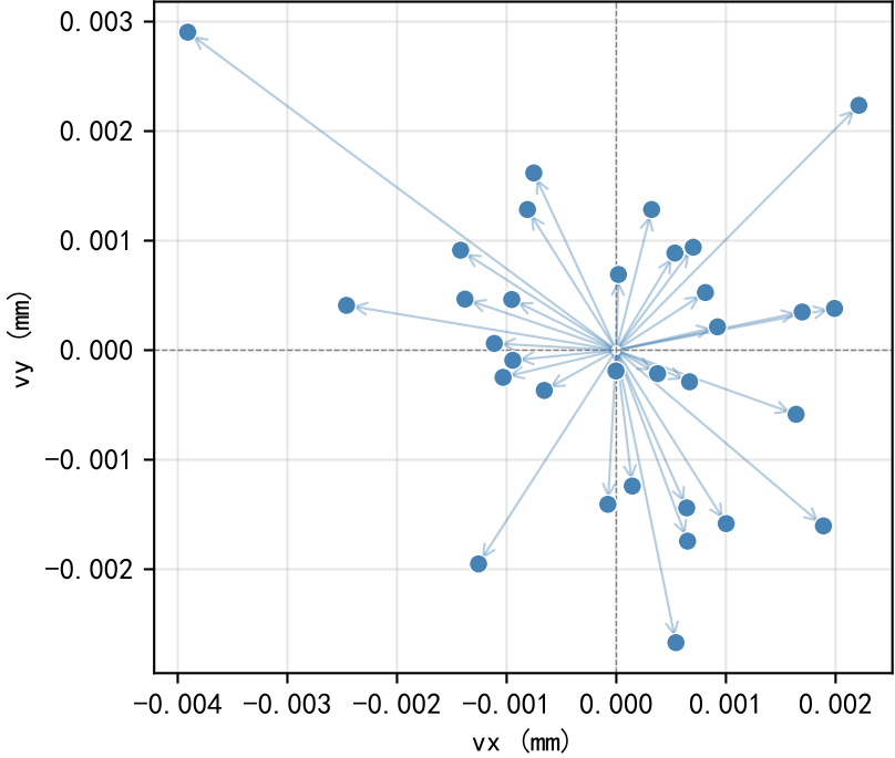
残差散点图 (sigma0=0.0018 mm)
