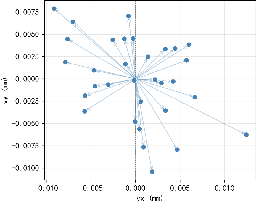
残差散点图 (sigma0=0.0066 mm)
