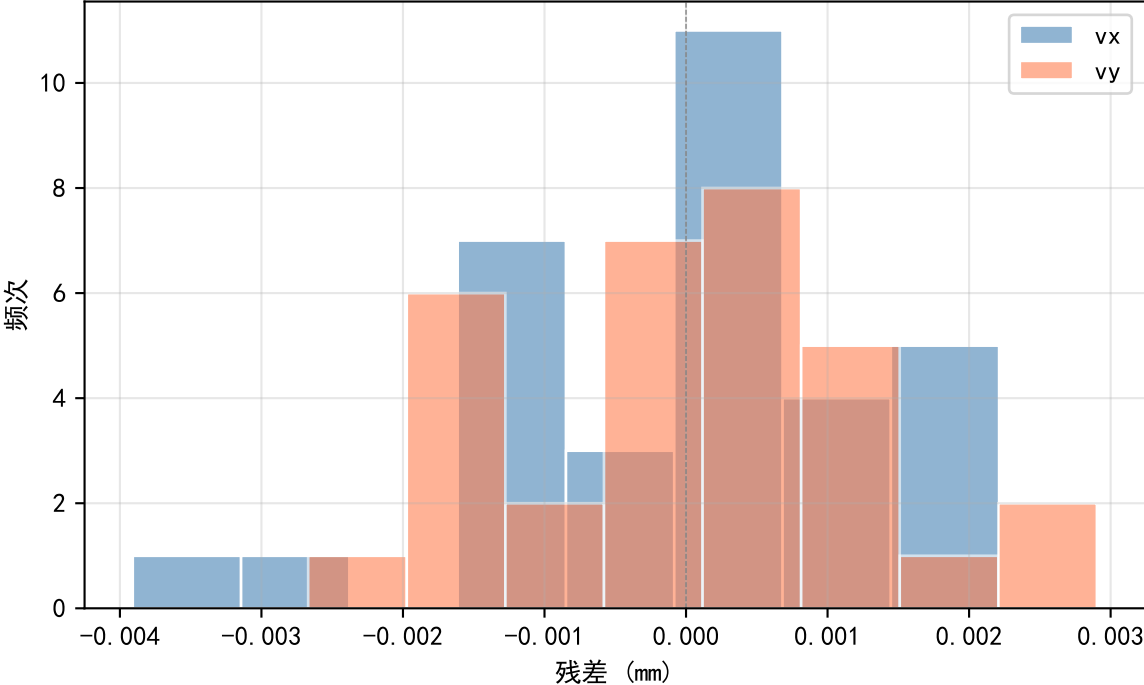
残差直方图
