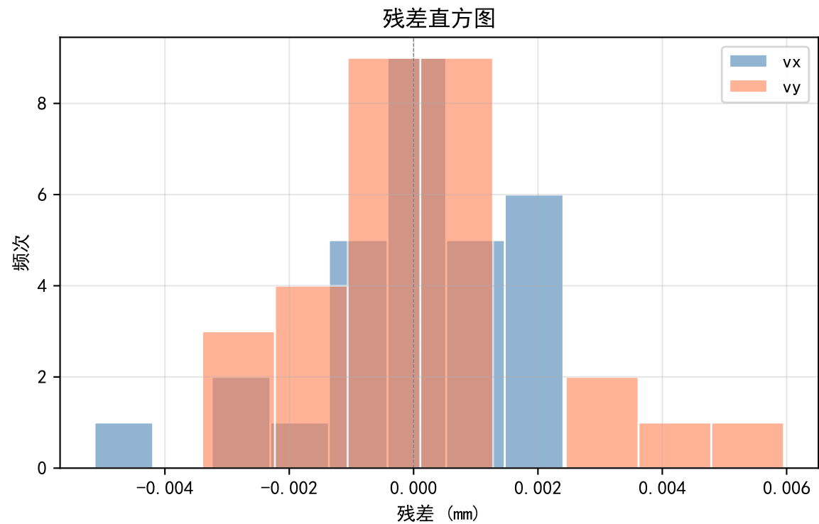
残差统计
