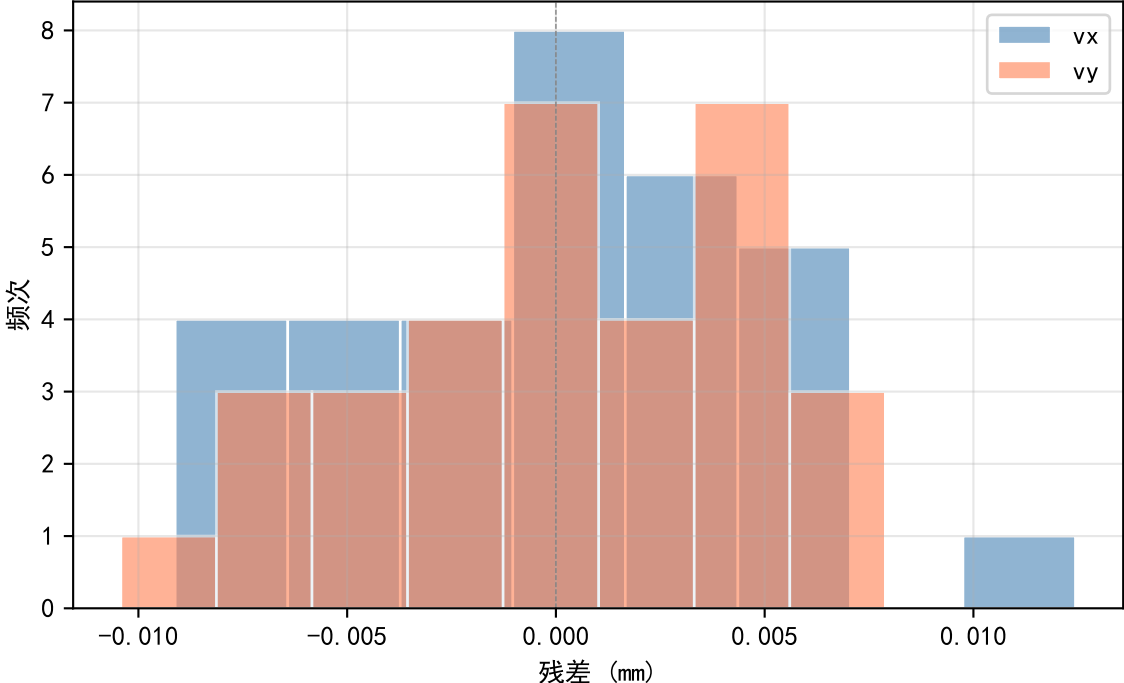
残差统计
