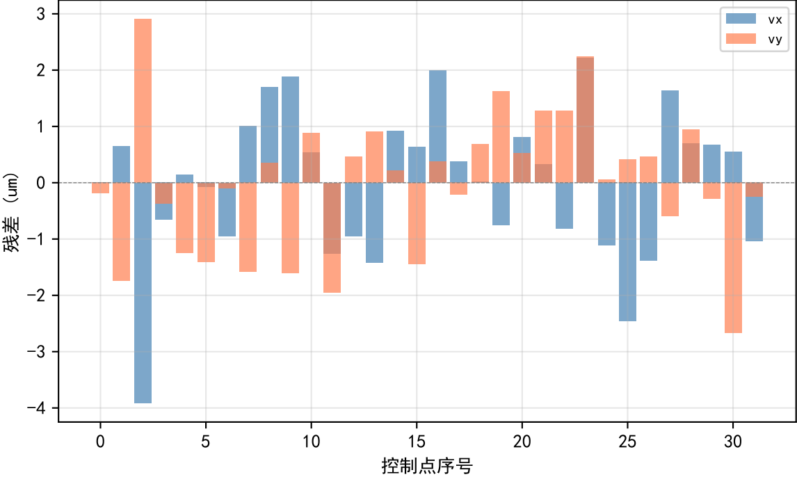
逐点残差
