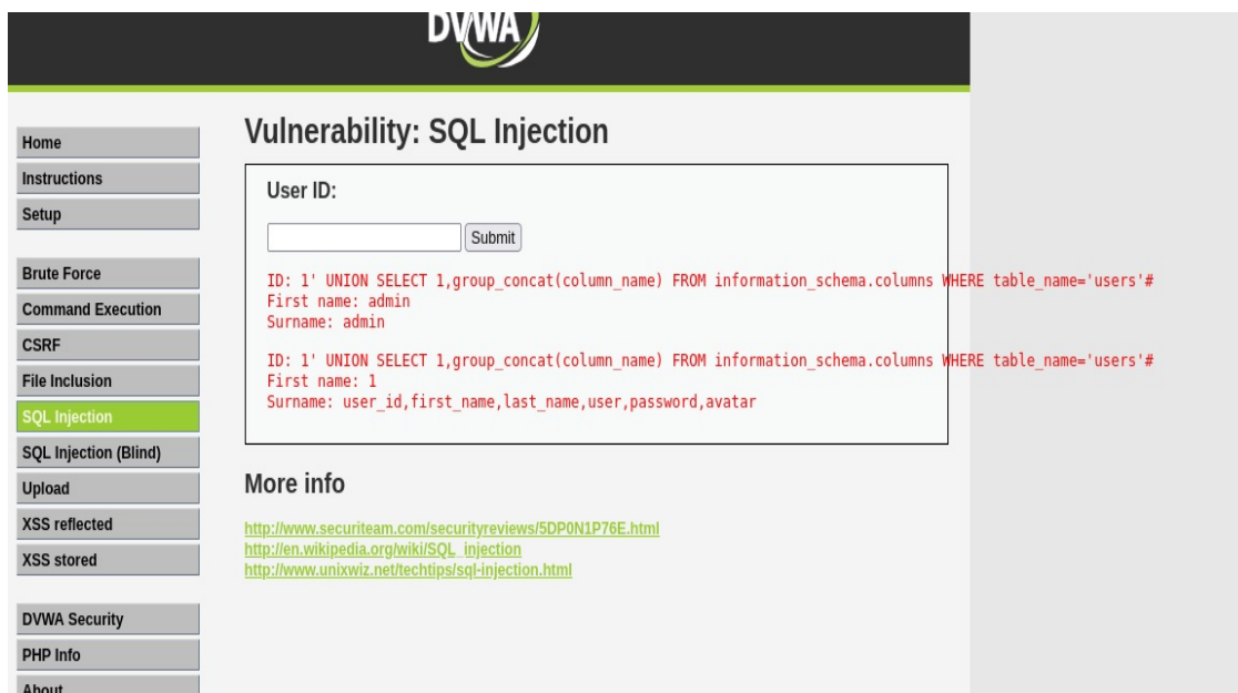
Figura 6 - Individuazione delle colonne della tabella users.
