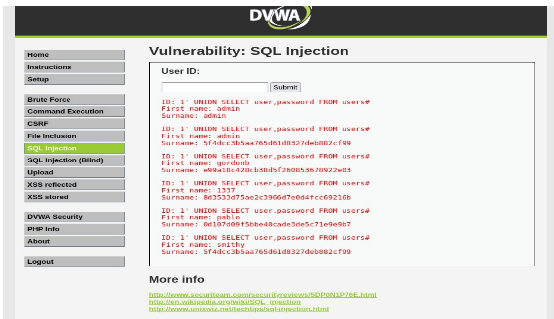
Figura 7 - Estrazione degli username e degli hash MD5.
