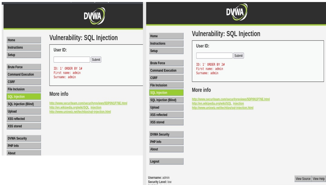
Figura 2 - Enumerazione delle colonne mediante ORDER BY.
