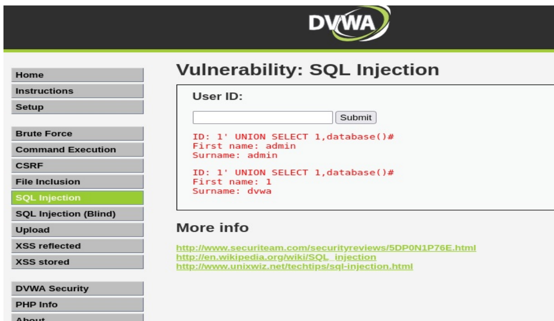
Figura 4 – Individuazione del database utilizzato (dvwa).
