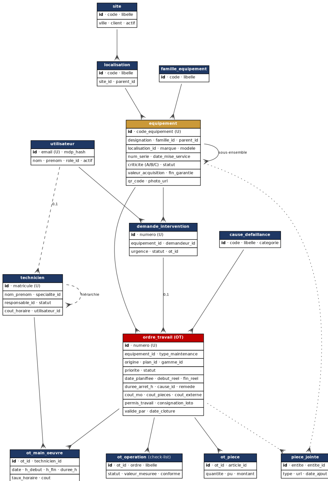
Figure 4 — Modèle de données cible : noyau actifs et exécution des interventions
