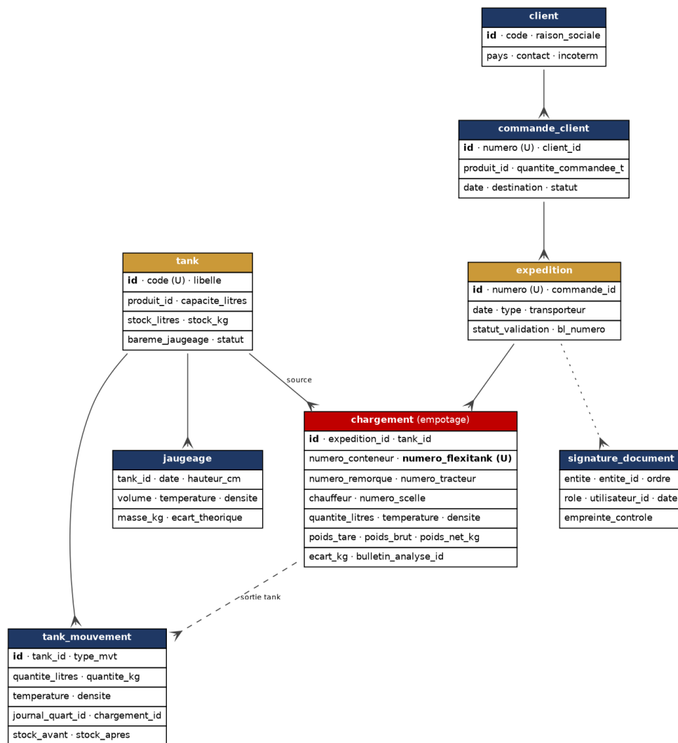
Figure 11 — Modèle de données du domaine Produit fini et expéditions
