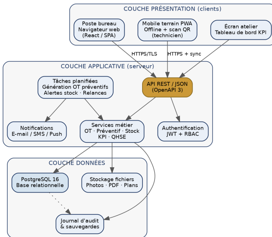
Figure 3 — Architecture applicative cible en trois couches
