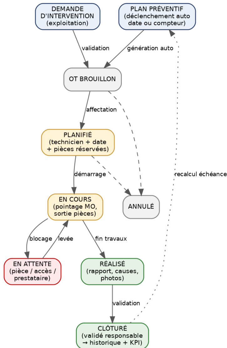
Figure 7 — Cycle de vie de l'ordre de travail
