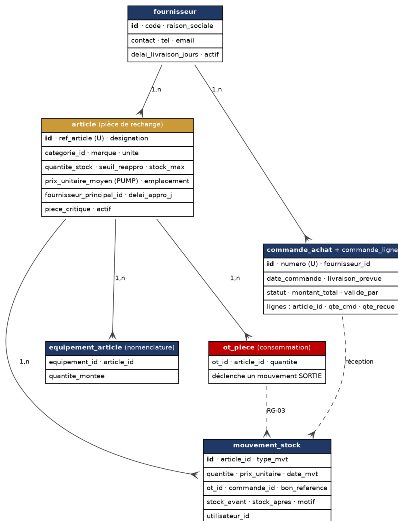
Figure 6 — Modèle cible : articles, mouvements de stock, fournisseurs et achats
