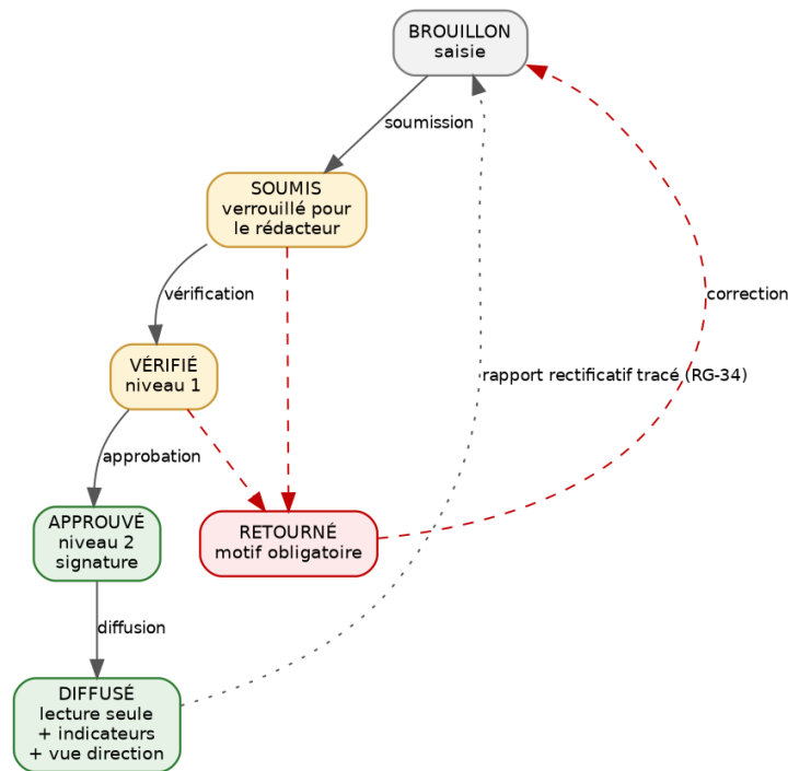
Figure 13 — Circuit générique de validation, commun à tous les documents
