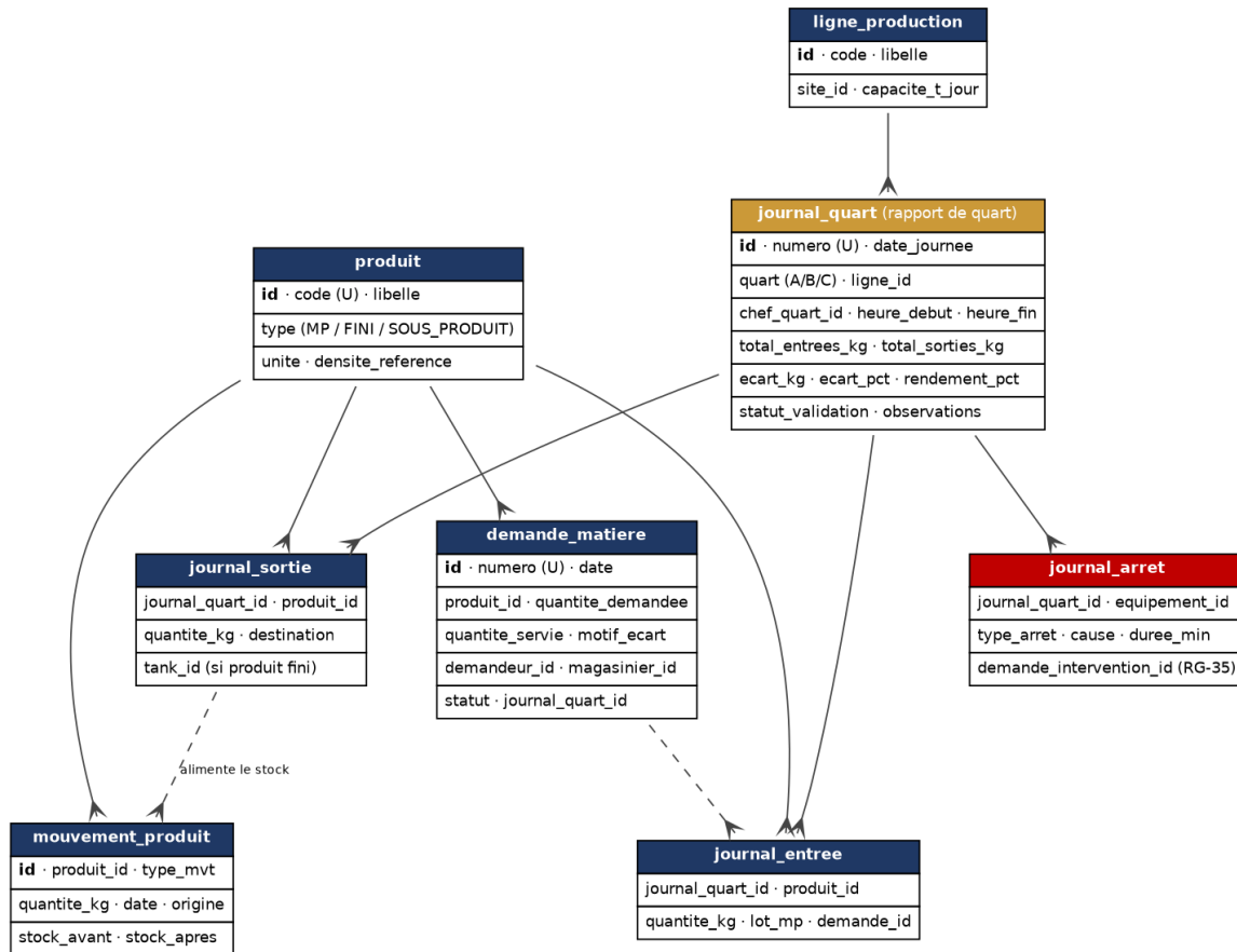
Figure 9 — Modèle de données du domaine Production
