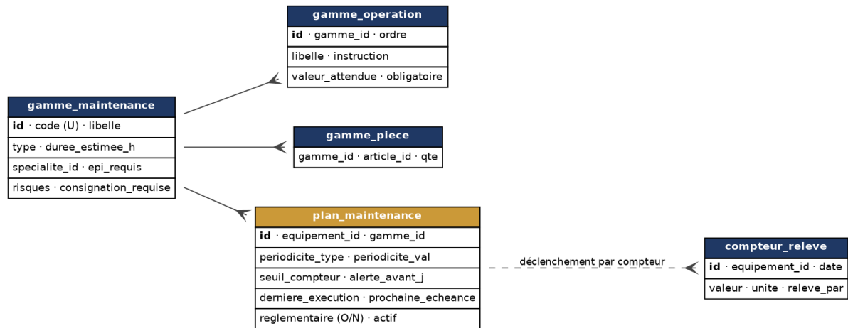
Figure 5 — Modèle cible : gammes, plans de maintenance préventive et compteurs
