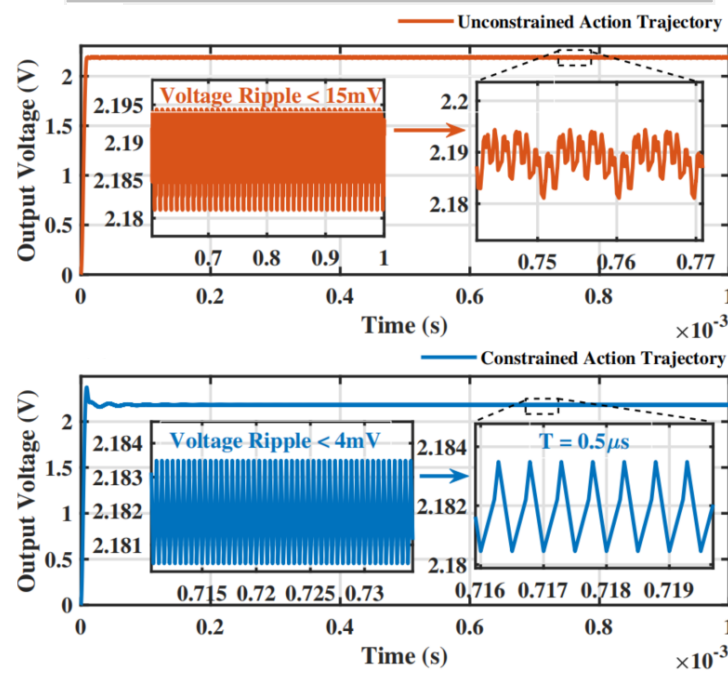
(d) Output Voltage Curve
